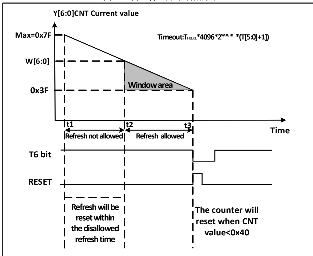
图 4-2 窗口看门狗的计数模式
