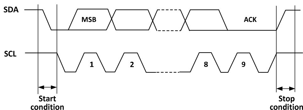
图 13-1 I2C 时序图
