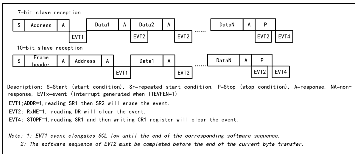
图 13-7 从接收器的传送序列图
