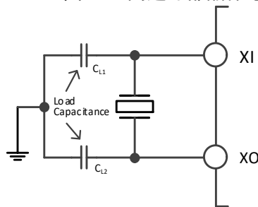
图 3-3 高速外部晶体电路
