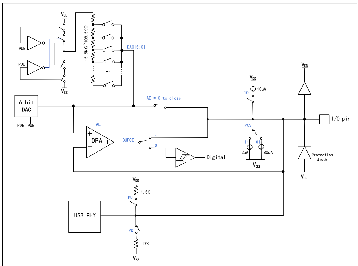
图 20-1 BC 接口结构图
