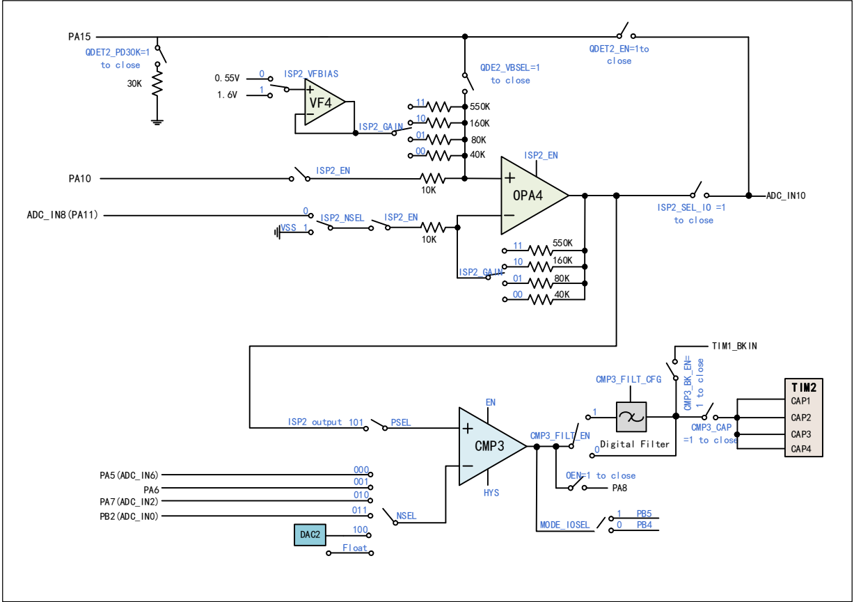
图 17-8 ISP2 结构图
