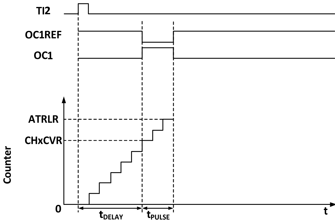
图 9-5 单脉冲的产生
