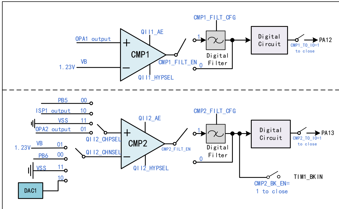
图 17-3 CMP1 和 CMP2 的结构图
