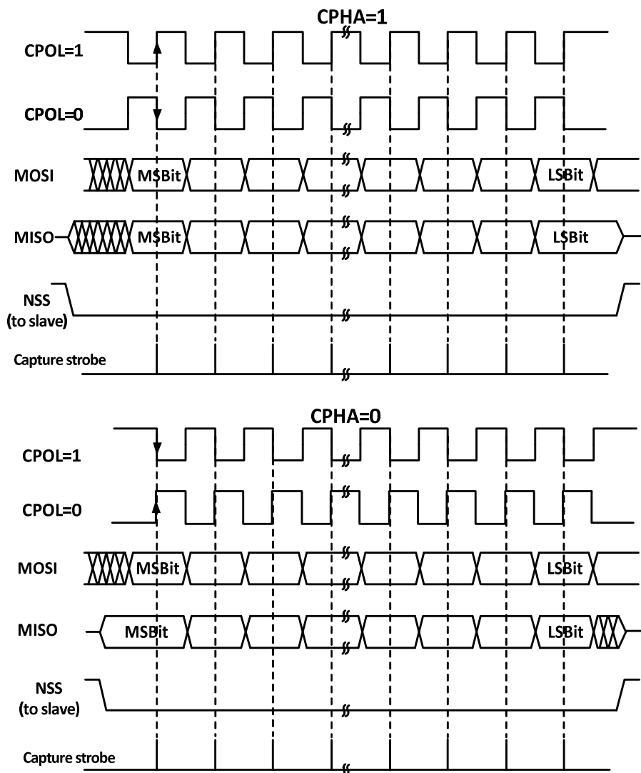
图 14-2 SPI 模式
