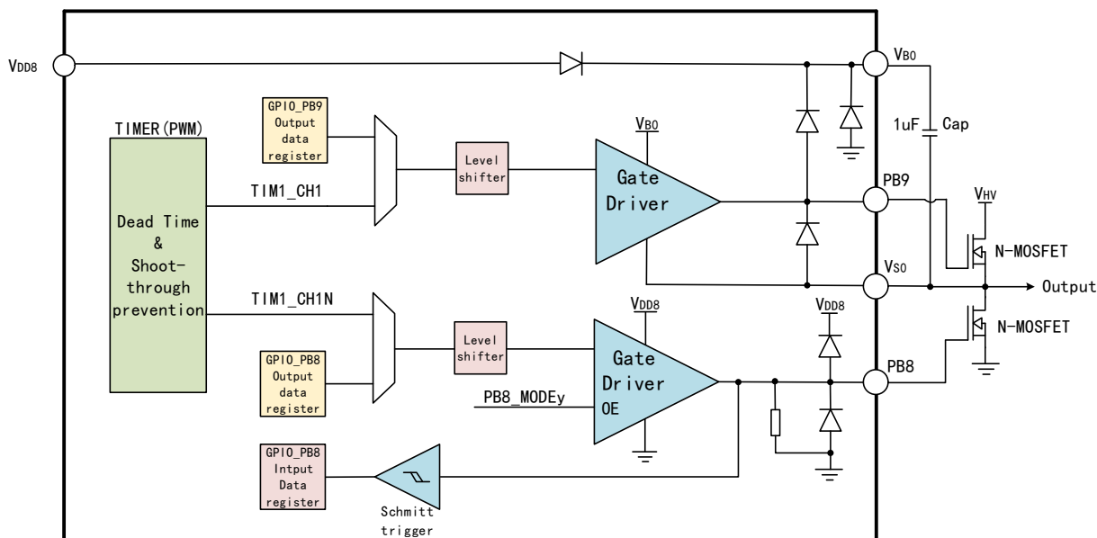
图 6-6 MV 的 GPIO 结构框图
