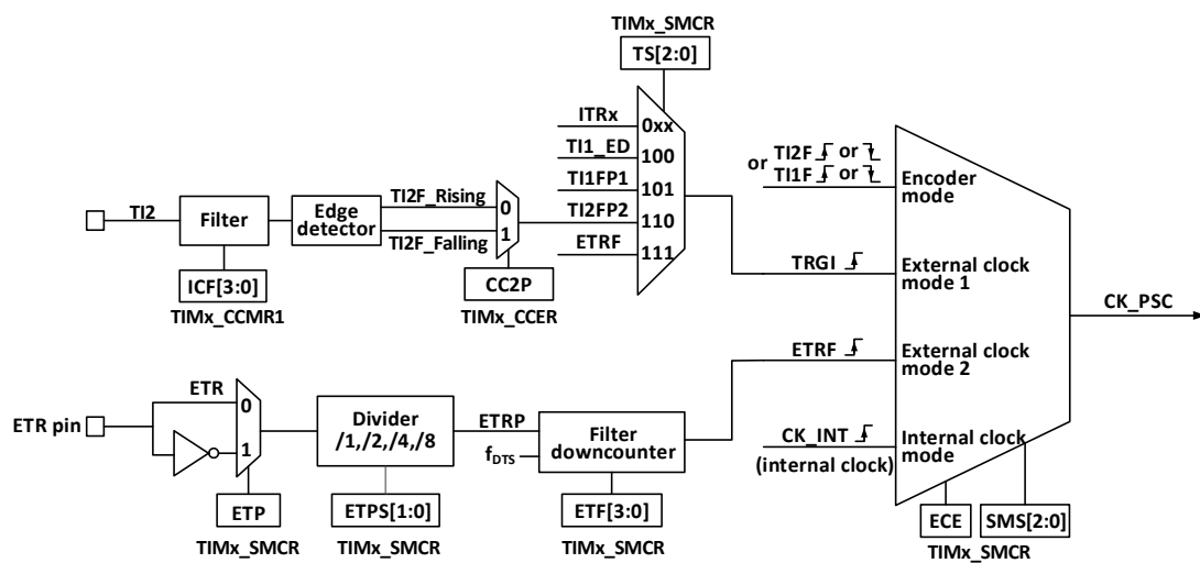
图 10-2 通用定时器 CK_PSC 来源框图
