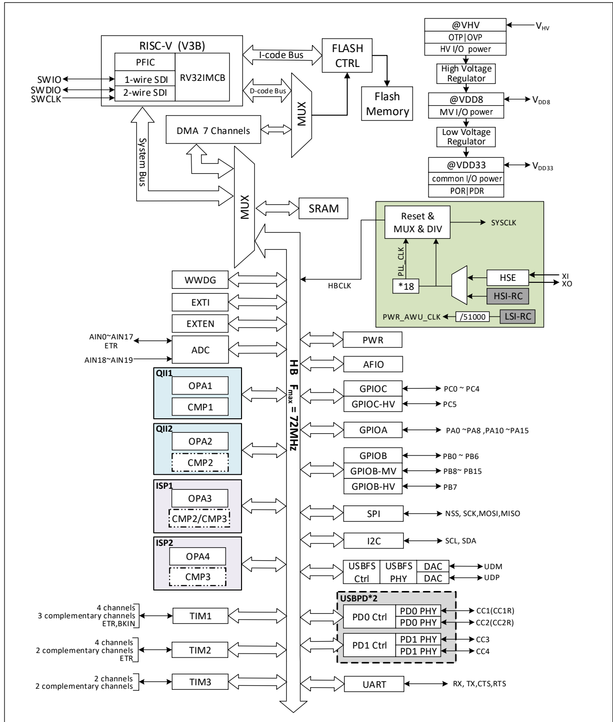
图 1-1 CH32M030 系统框图
