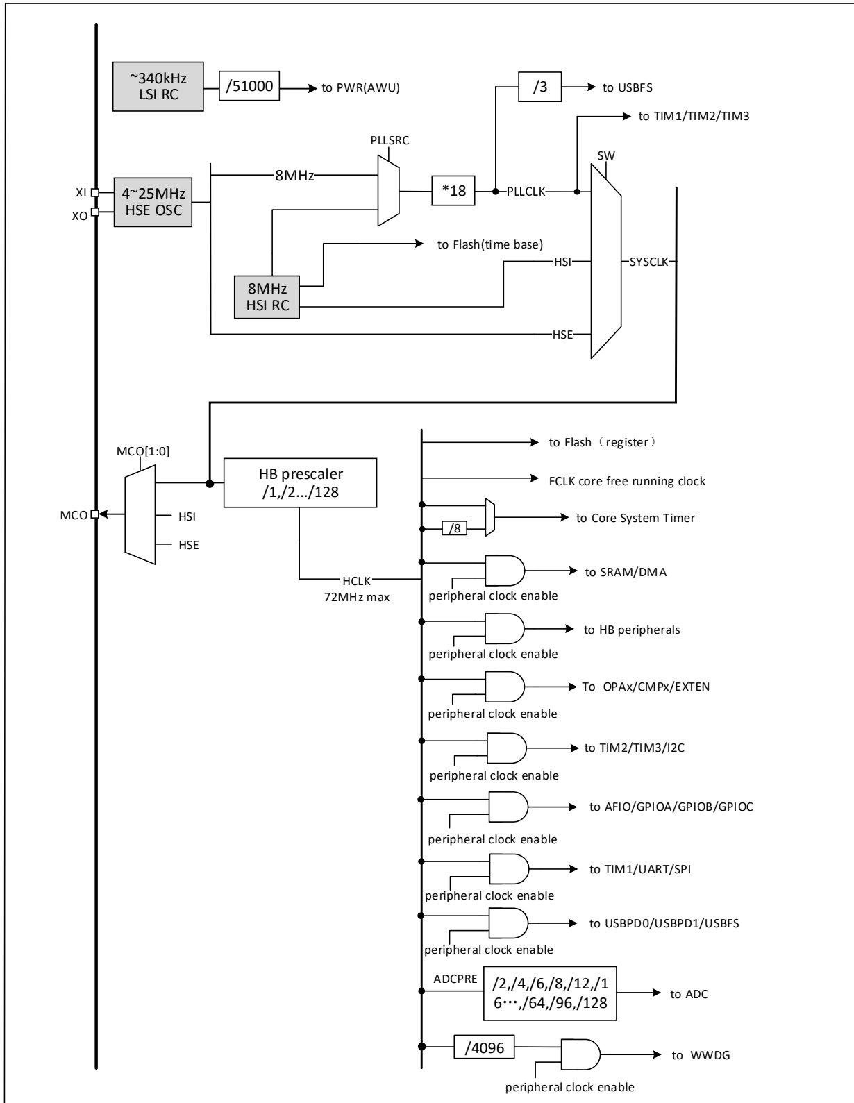
图 3-2 时钟树结构
