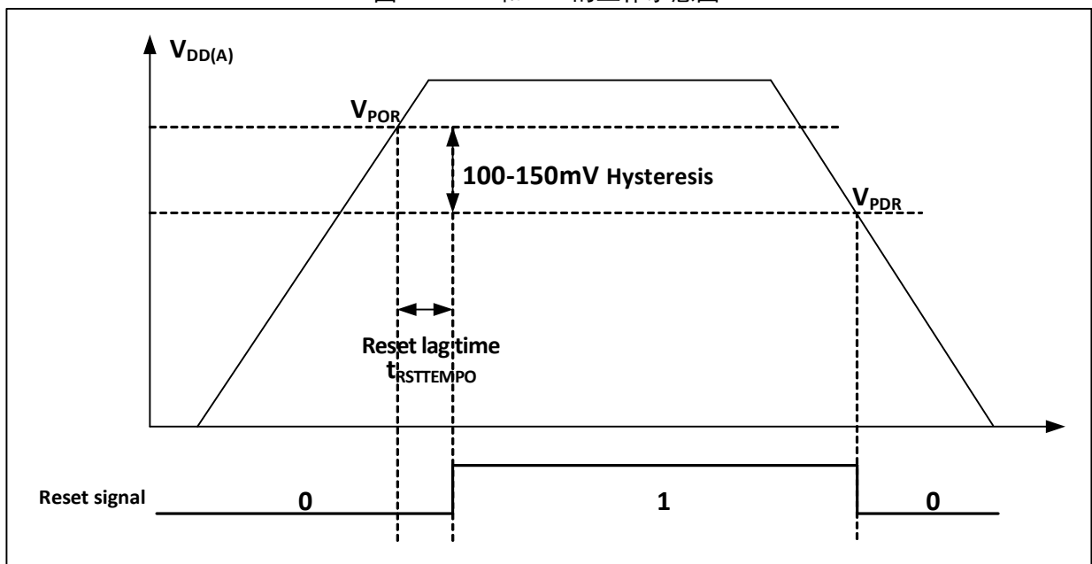
图 2-1 POR 和 PDR 的工作示意图
