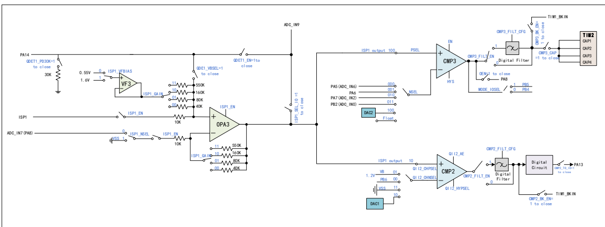
图 17-7 ISP1 结构图
