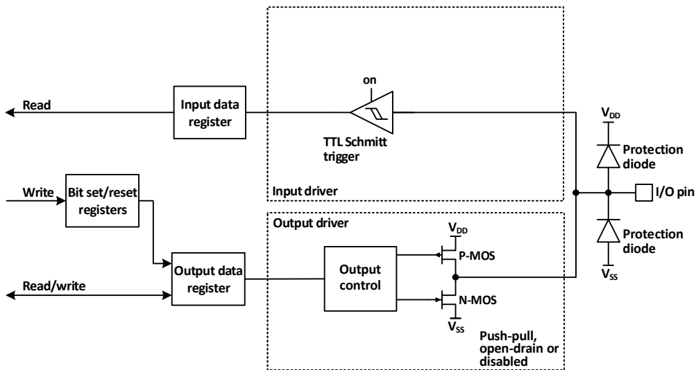
图 6-3 GPIO 模块输出配置结构框图
