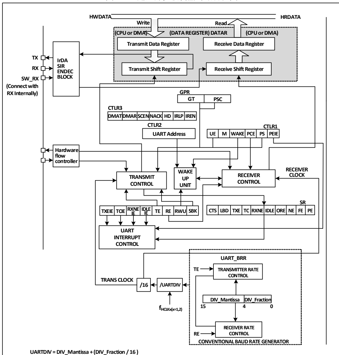
图 12-1 通用异步收发器的结构框图
