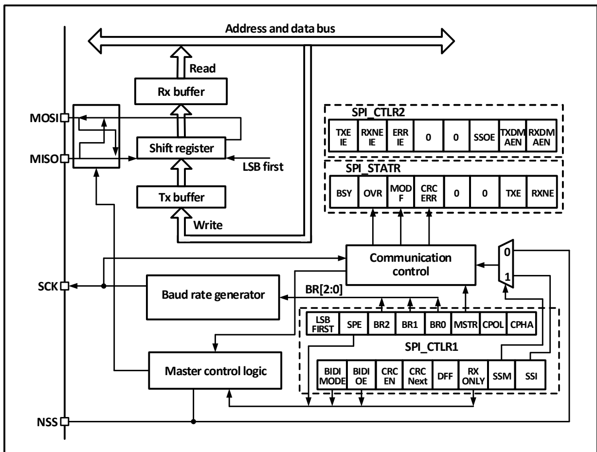
图 14-1 串行外设总线结构框图
