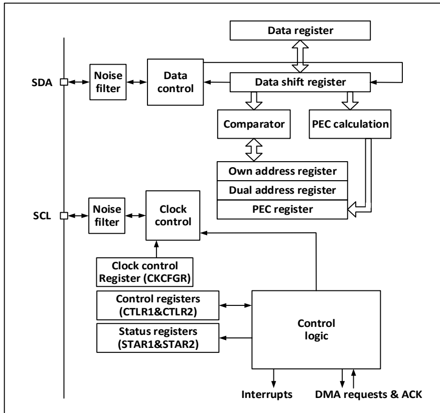
图 13-2 I2C 功能框图
