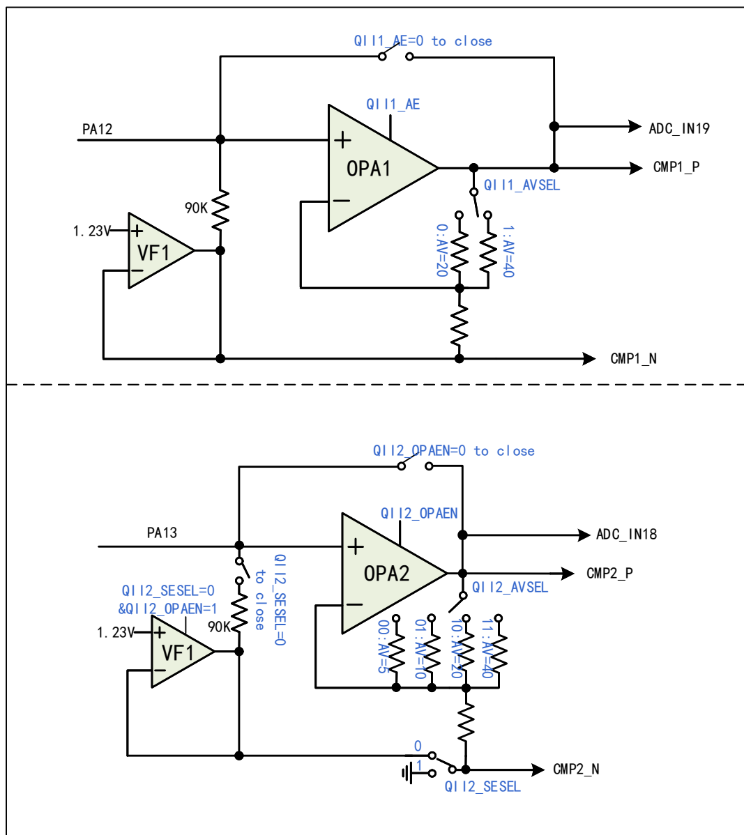
图 17-1 OPA1 和 OPA2 的结构图
