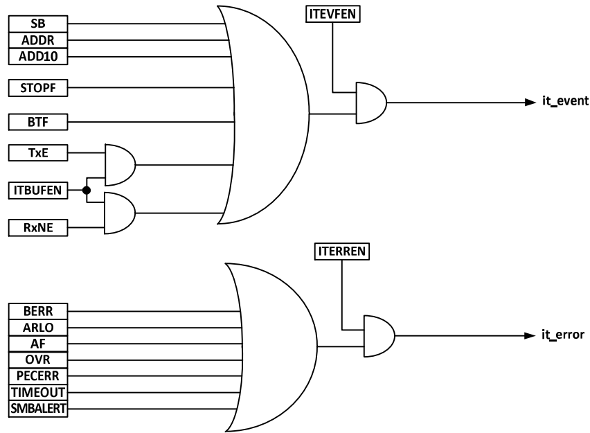
图 13-8 I2C 中断请求
