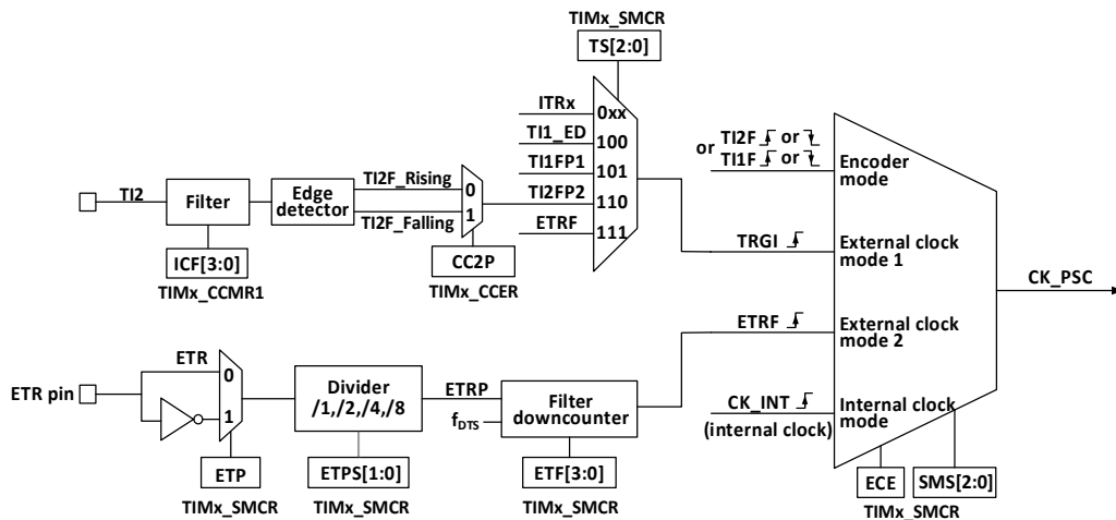
图 9-2 高级定时器的 CK_PSC 来源框图
