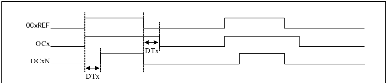
图 11-4 互补输出和死区
