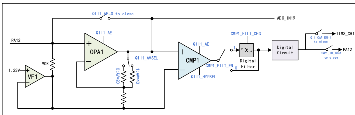
图 17-5 QII1 结构图
