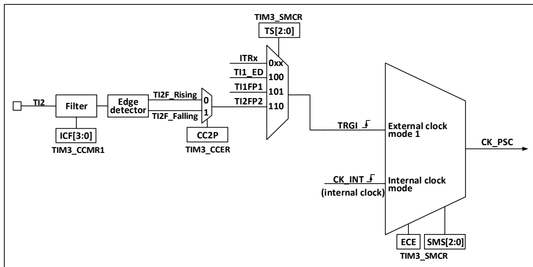
图 11-2 精简定时器 CK_PSC 来源框图
