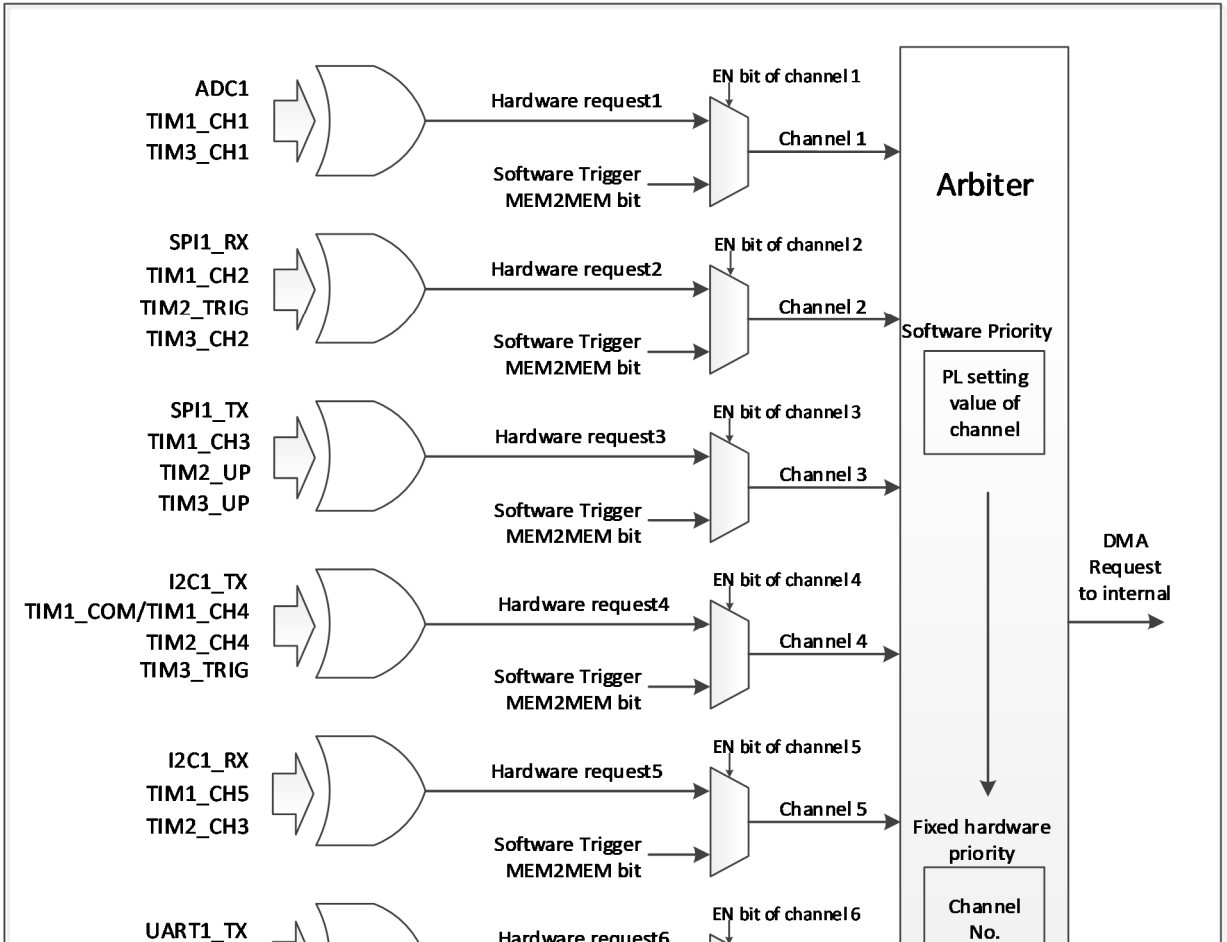
图 7-1 DMA 请求映像
