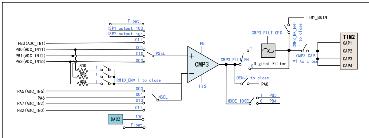
图 17-4 CMP3 结构图
