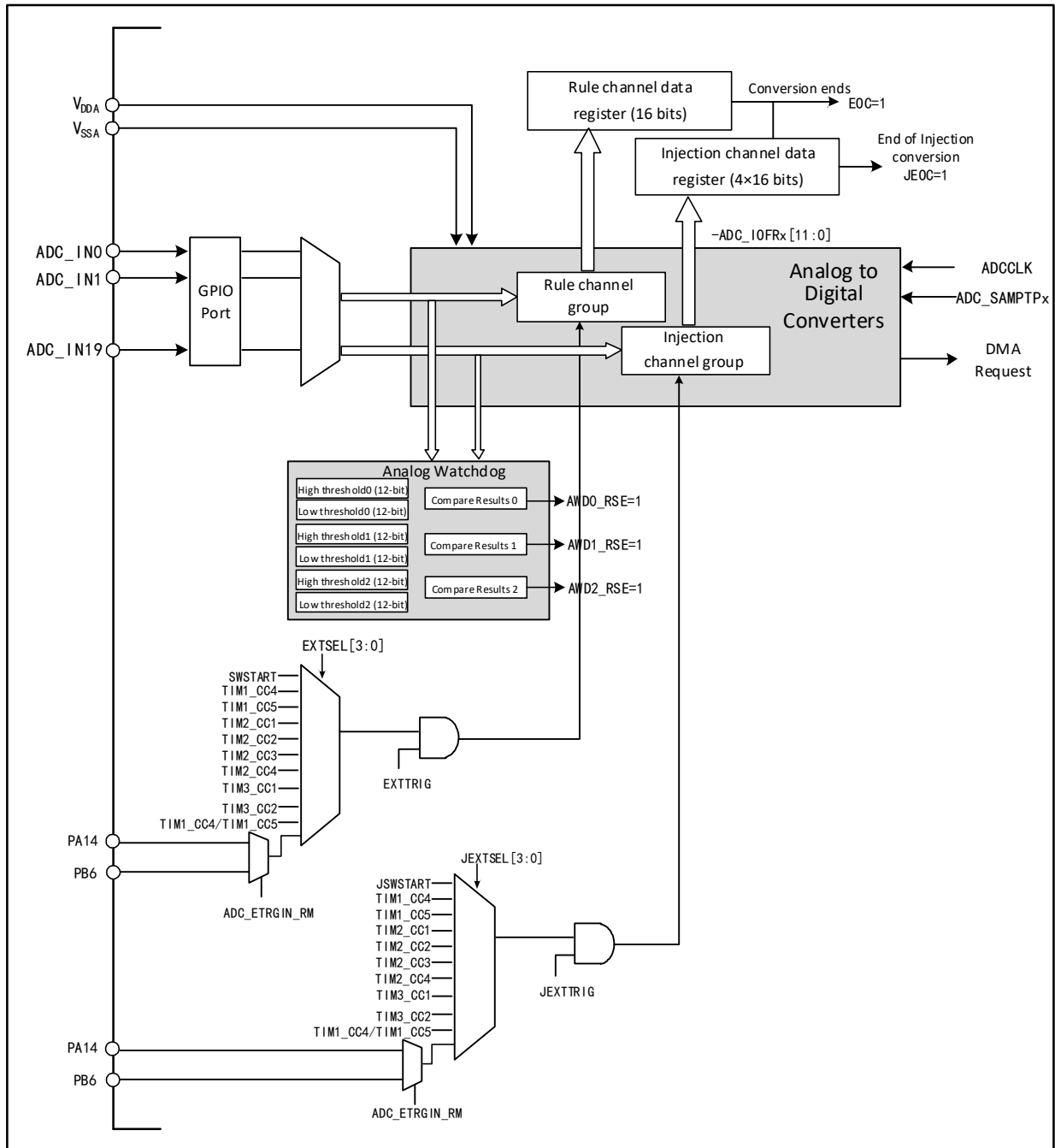
图 8-1 ADC 模块框图
