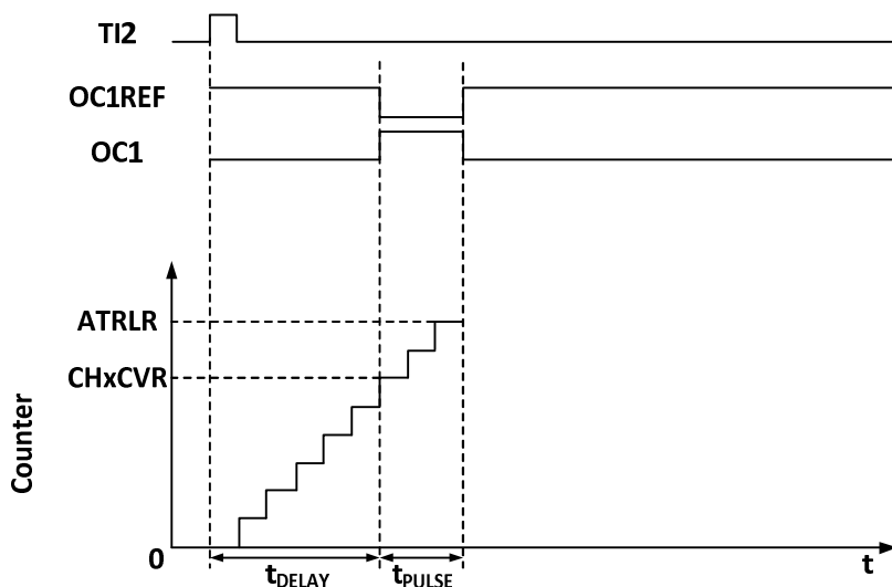
图 11-5 事件产生和脉冲响应
