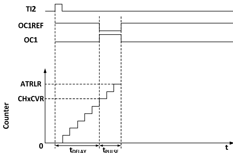
图 10-4 事件产生和脉冲响应
