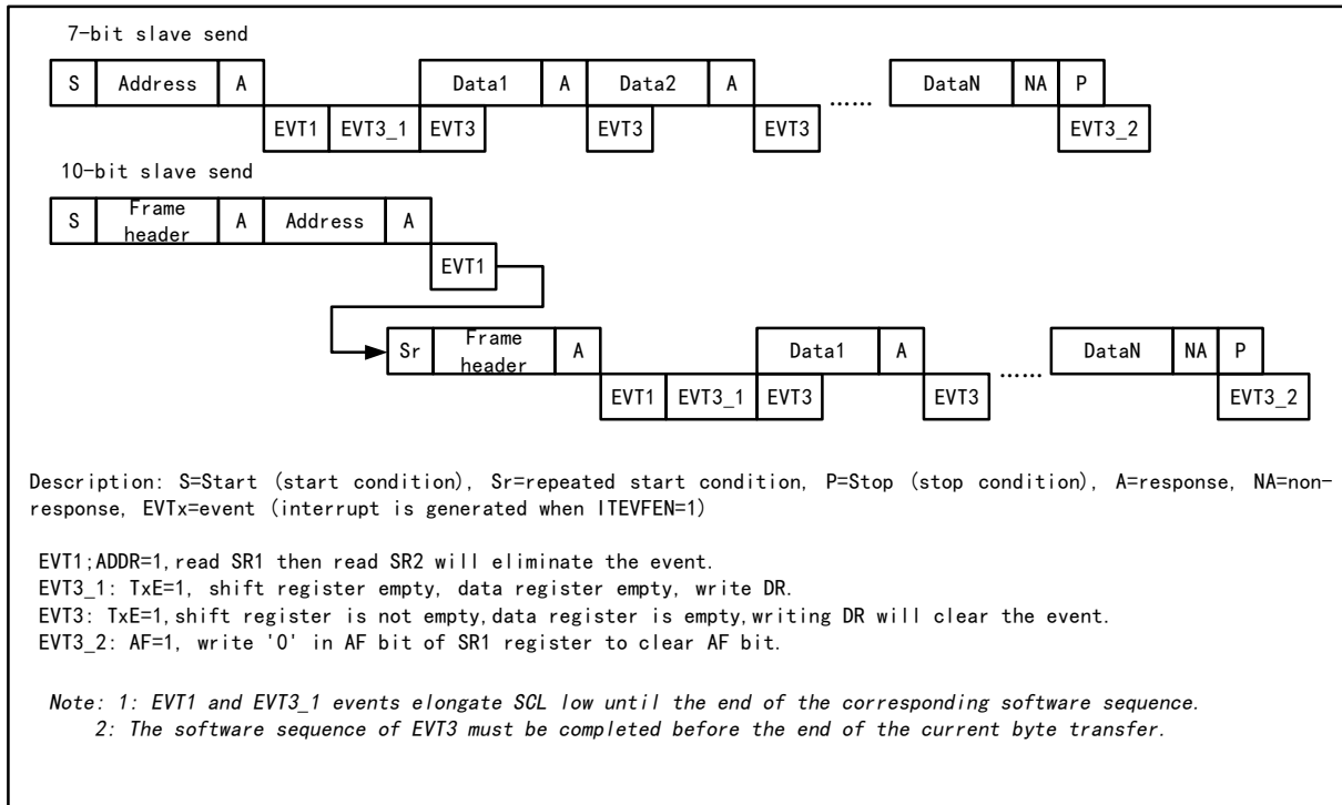
图 13-6 从发送器的传送序列图
