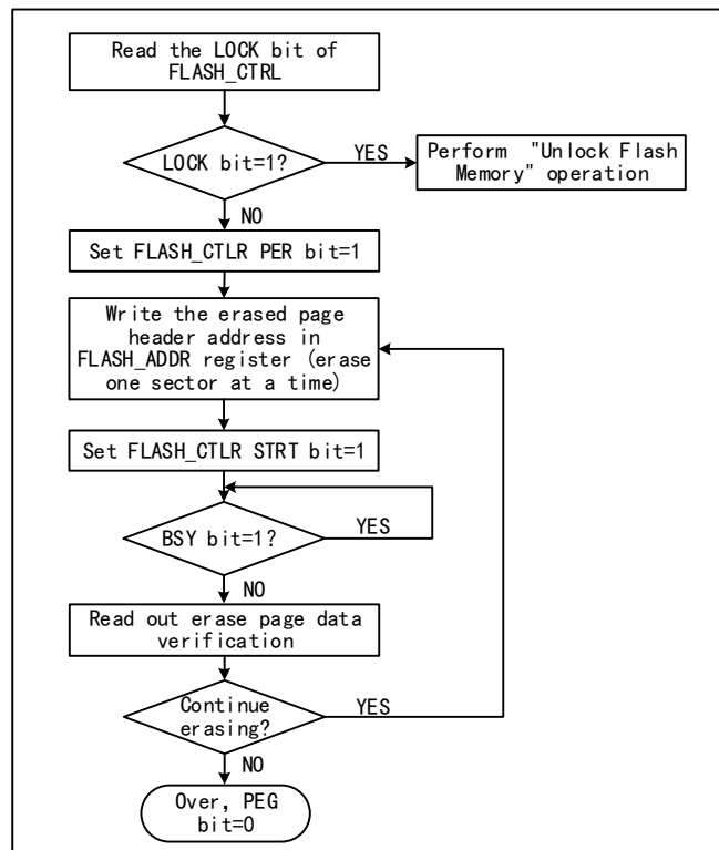
图 19-1 FLASH 页擦除
