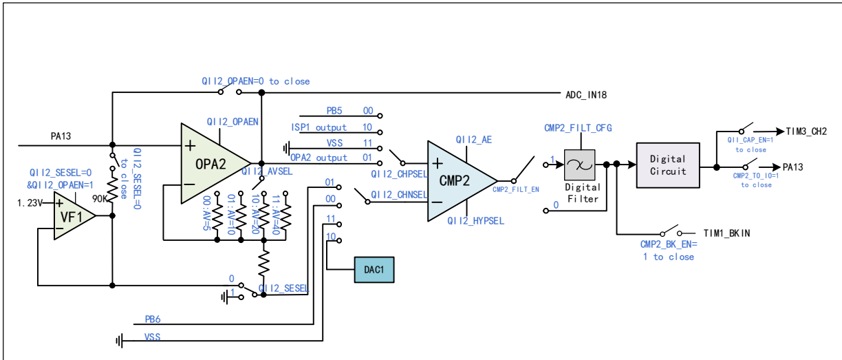
图 17-6 Q112 结构图
