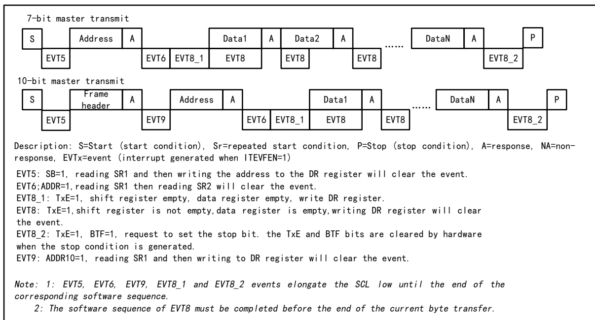
图 13-4 主发送器传送序列图
