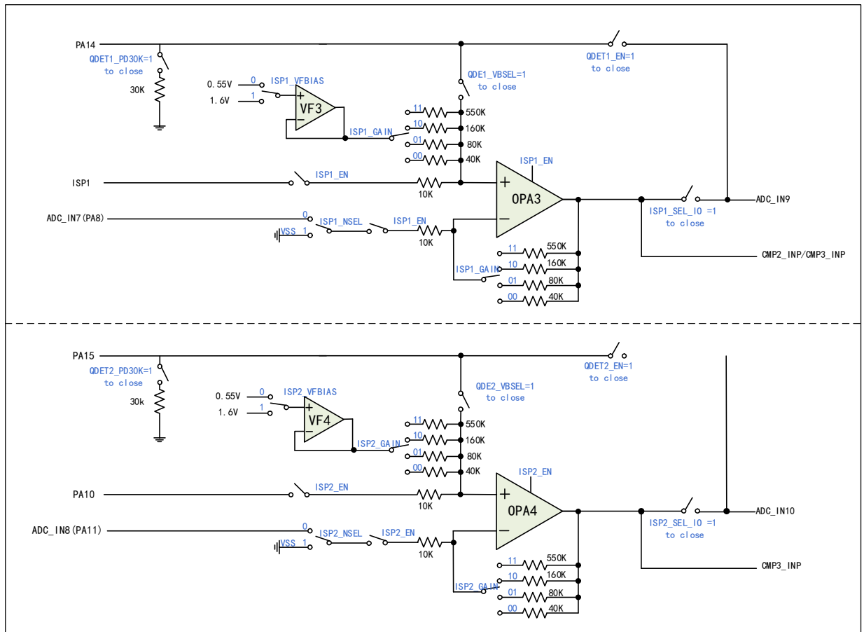
图 17-2 OPA3 和 OPA4 的结构图
