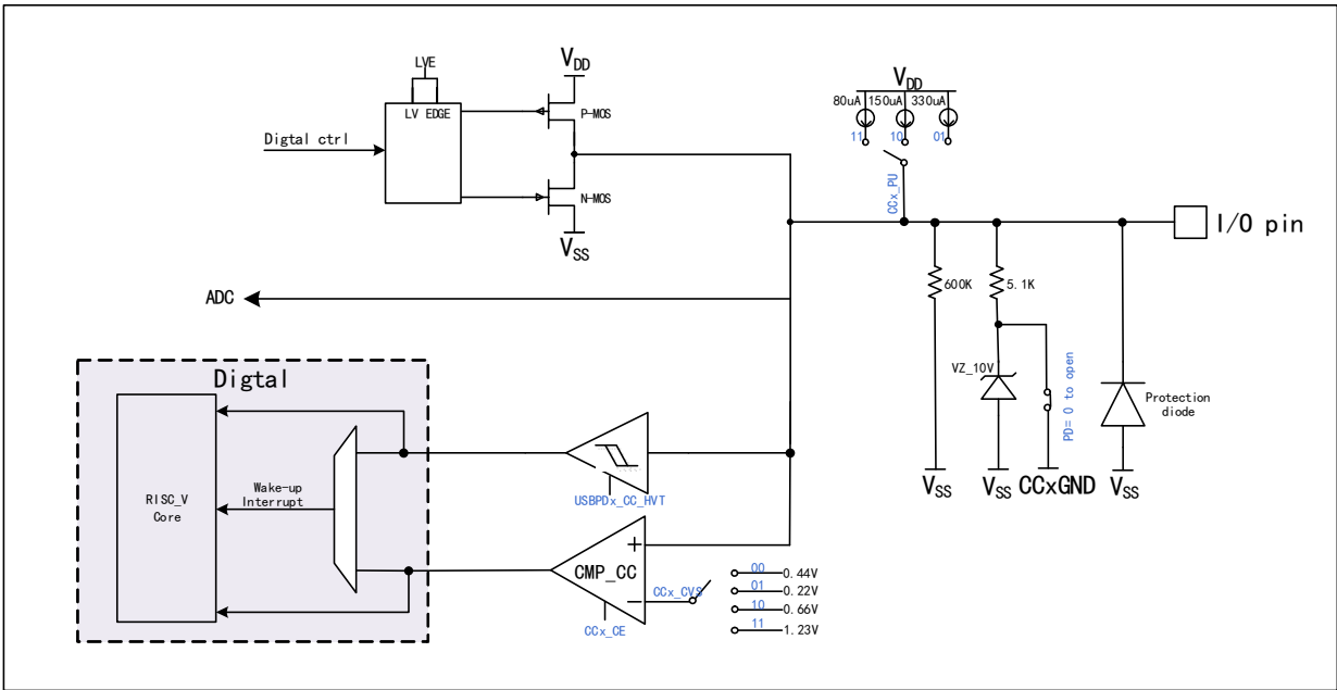
图 15-1 CC 端口结构图
