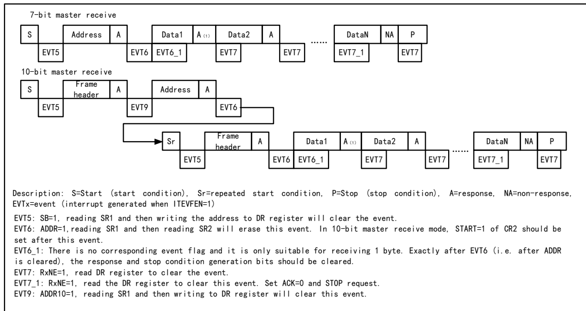
图 13-5 接收器传送序列图
