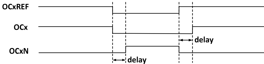
图 9-4 互补输出和死区
