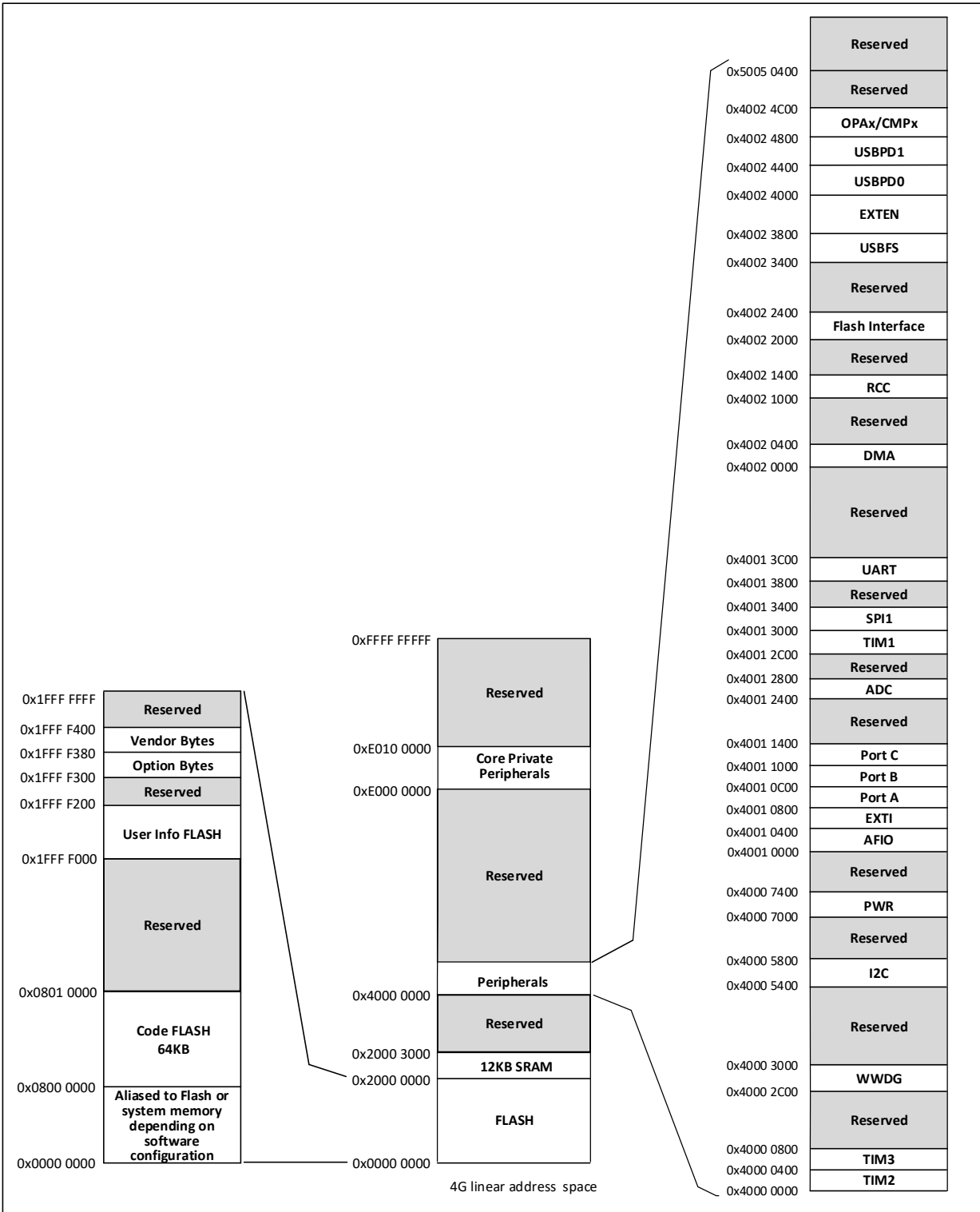
图 1-2 CH32M030 存储映像
