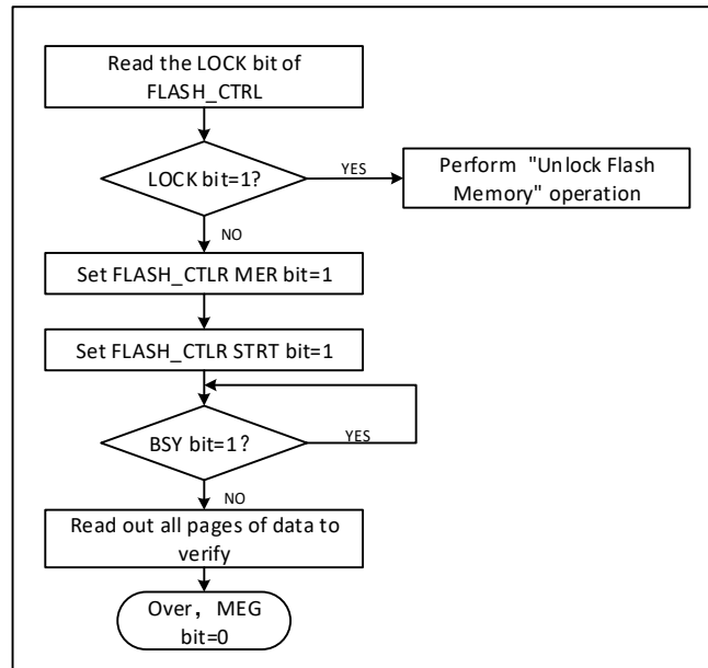
图 19-2 FLASH 整片擦除
