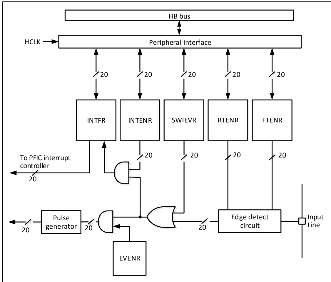
图 5-1 外部中断 (EXTI) 接口框图
