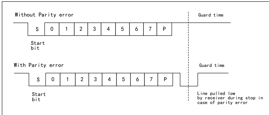
图 14-4（未）发生奇偶校验错误示意图
