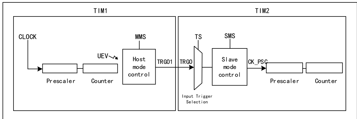
图 12-10 主/从定时器示例
