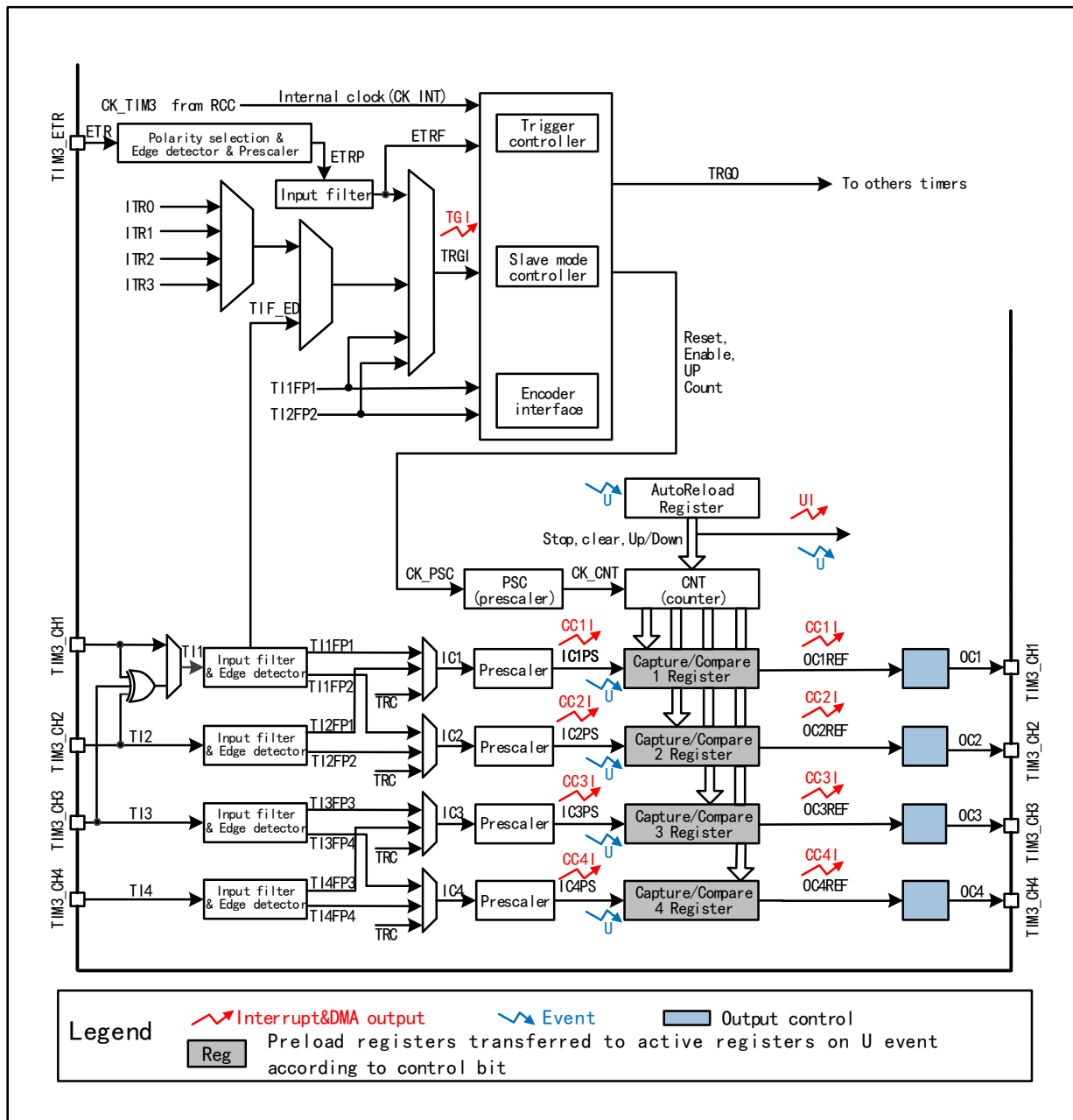
图 13-1 通用定时器的结构框图
