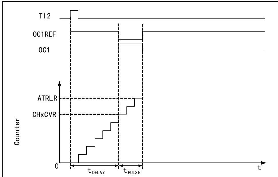
图 12-5 单脉冲的产生
