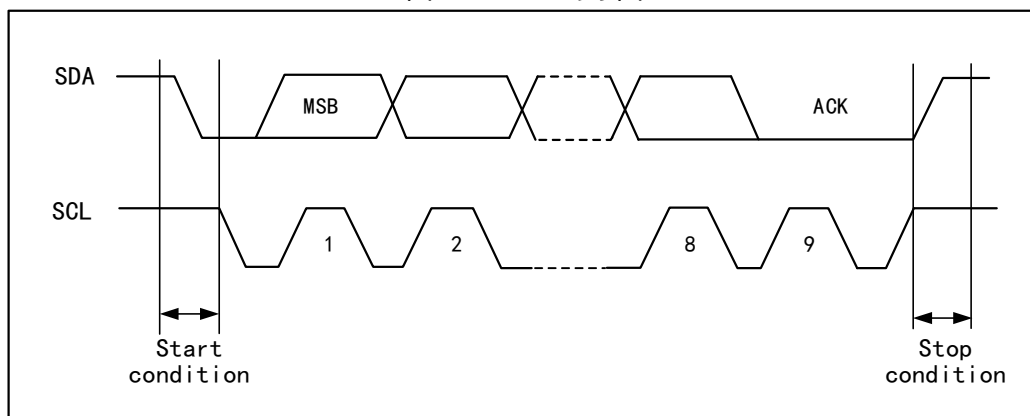
图 15-1 I2C 时序图
