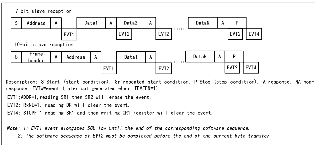
图 15-6 从接收器的传送序列图
