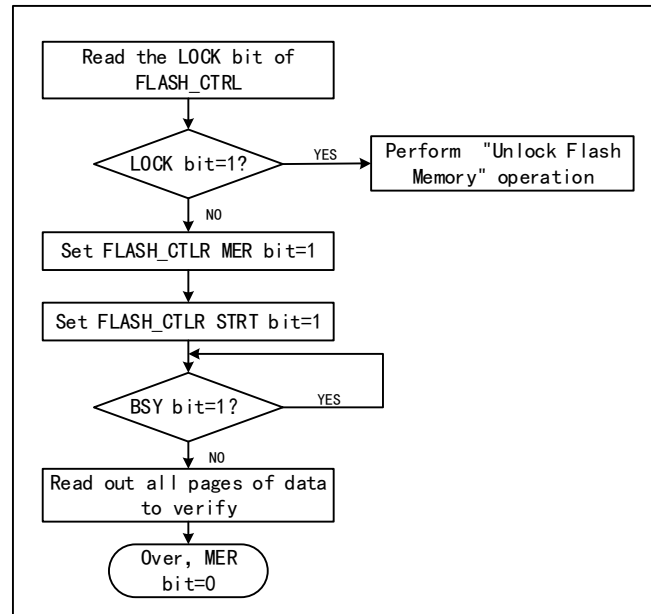
图 20-2 FLASH 整片擦除
