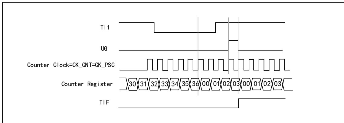
图 12-6 复位模式下的控制电路
