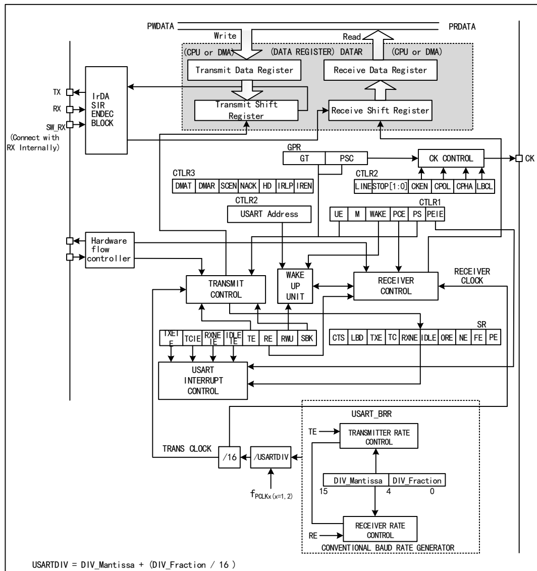
图 14-1 通用同步/异步收发器的结构框图
