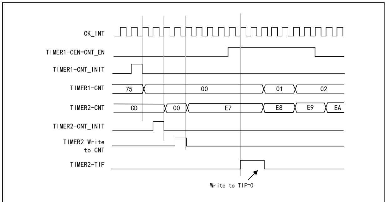
图 12-14 使用定时器 1 的使能信号触发定时器 2
