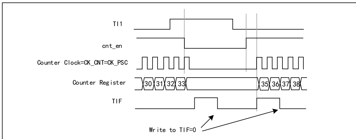
图 13-6 门控模式下的控制电路
