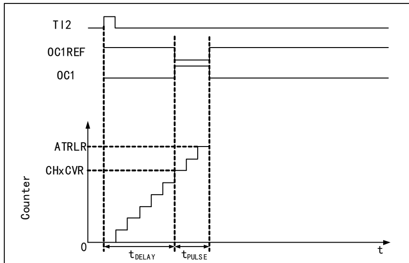
图 13-4 事件产生和脉冲响应
