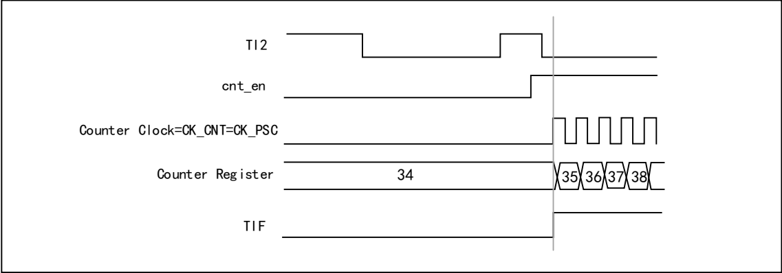
图 13-7 触发模式下的控制电路
