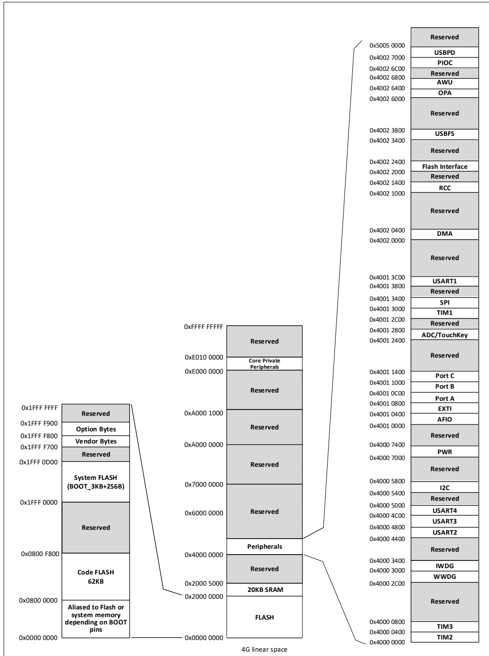
图 1-2 存储映像
