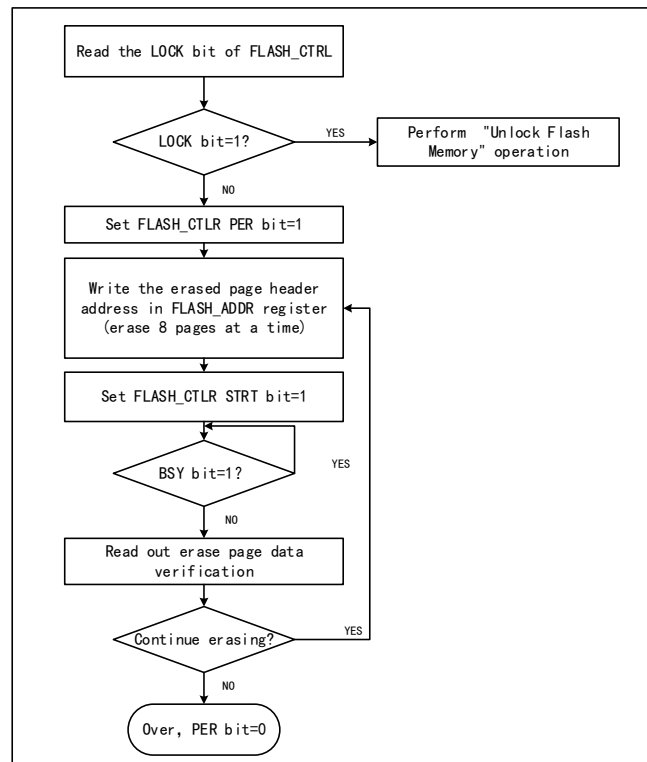
图 20-1 FLASH 页擦除
