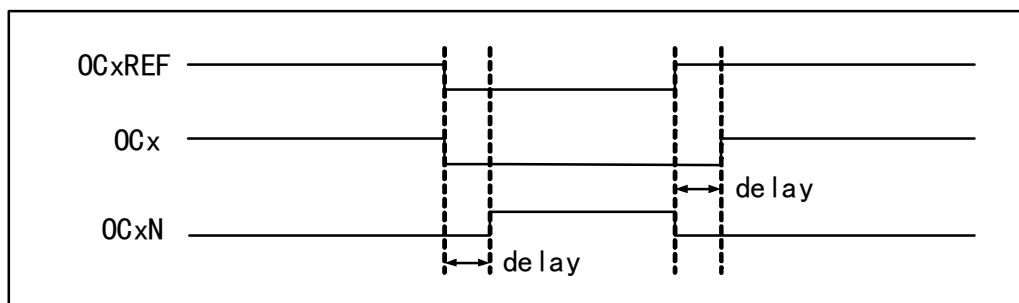
图 12-4 互补输出和死区
