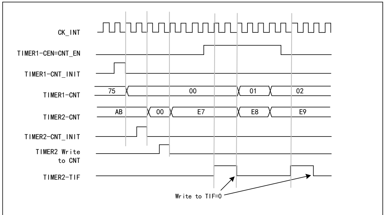
图 12-12 使用定时器 1 的使能信号对定时器 2 实施门控控制
