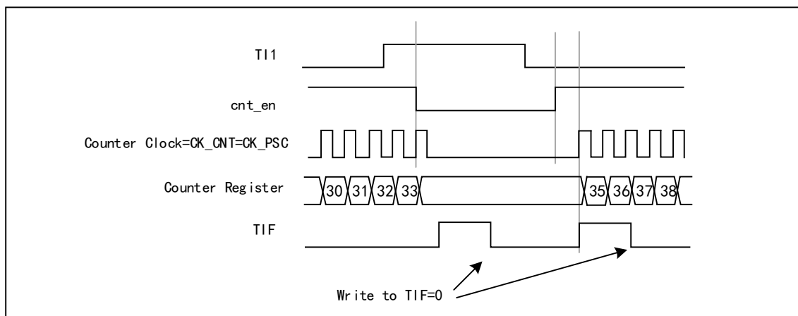
图 12-7 门控模式下的控制电路
