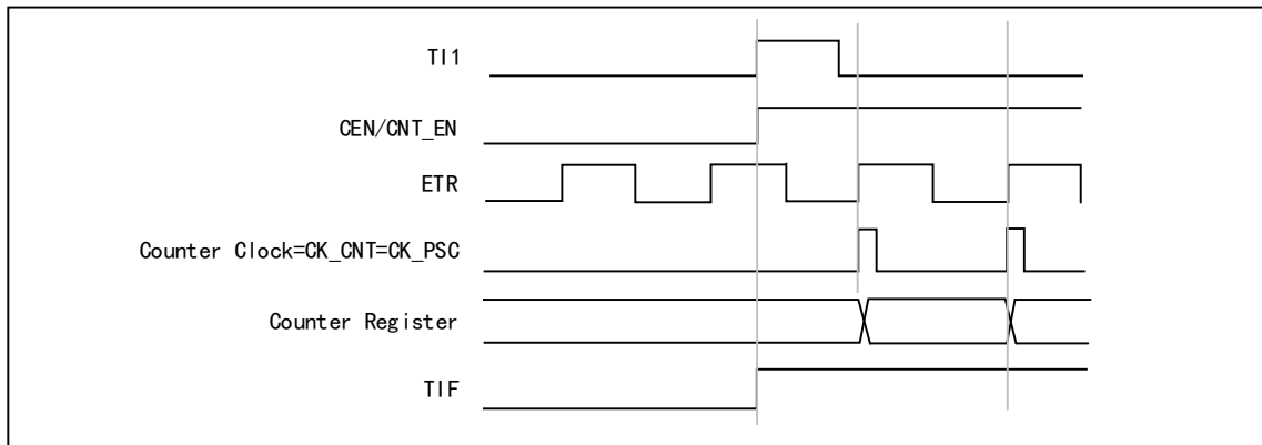
图 12-9 外部时钟模式 2+触发模式下的控制电路
