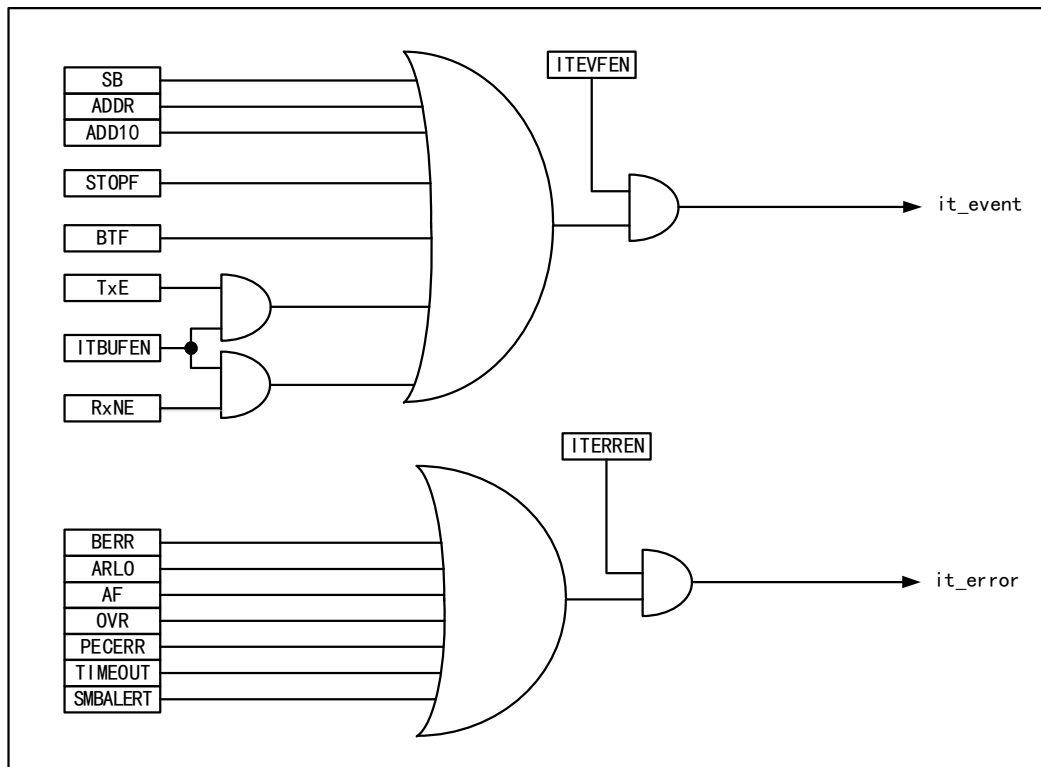
图 15-7 I2C 中断请求
