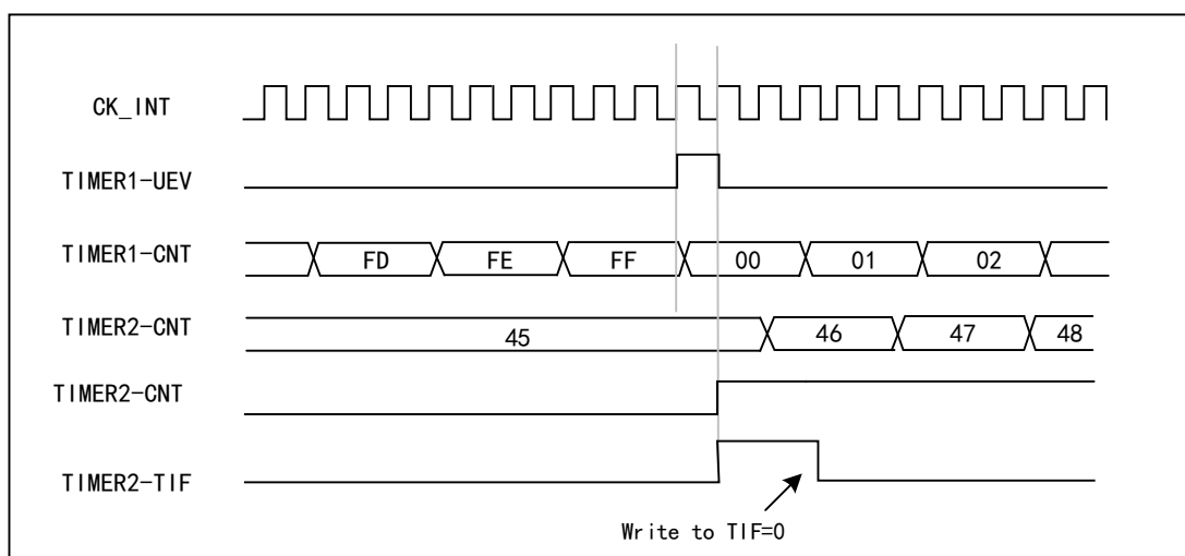
图 12-13 使用定时器 1 的更新事件触发定时器 2
