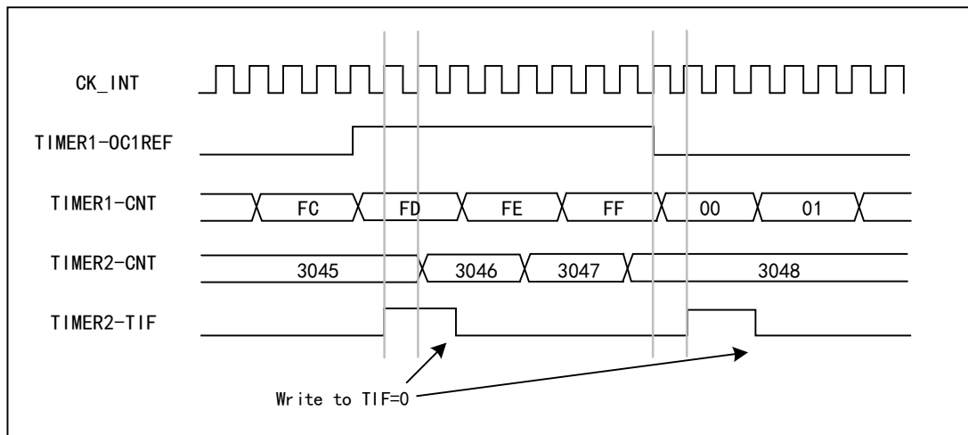
图 12-11 使用定时器 1 的 OC1REF 对定时器 2 实施门控控制
