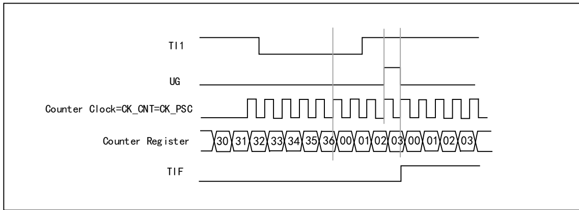
图 13-5 复位模式下的控制电路
