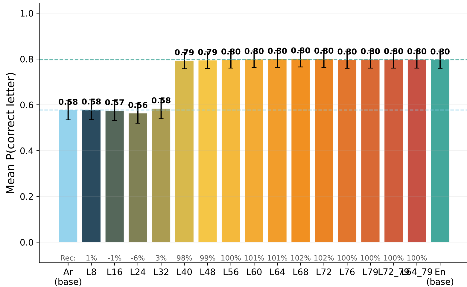
Llama-3.3-70B
