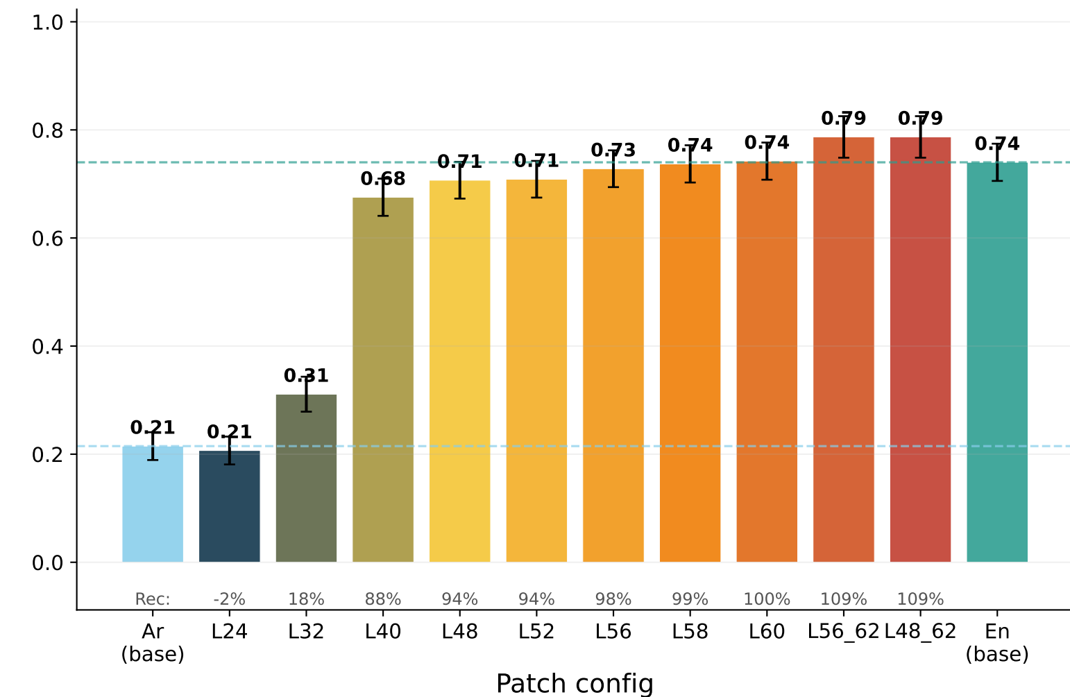
MedGemma-27B
