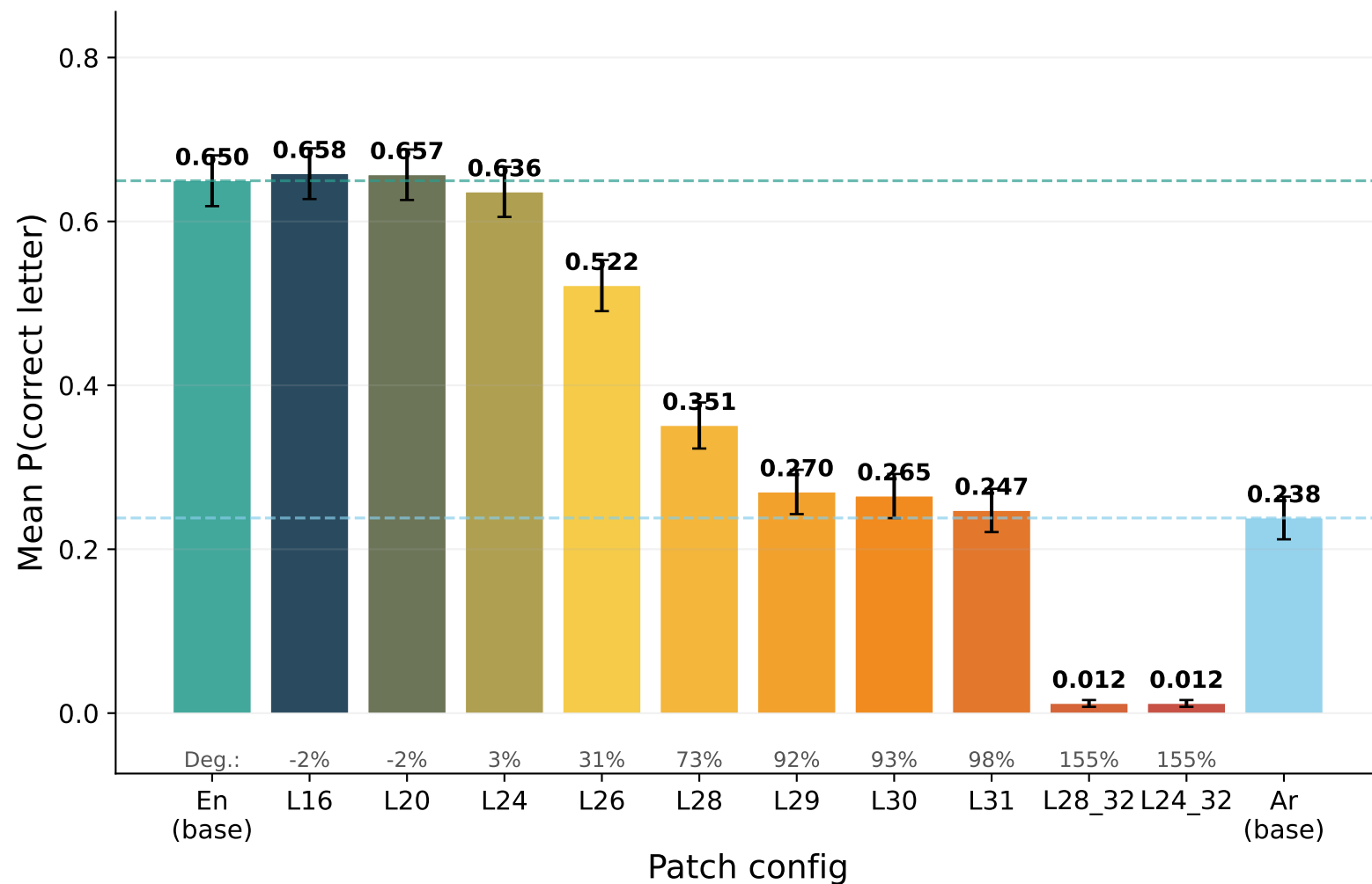
ALLaM-7B
