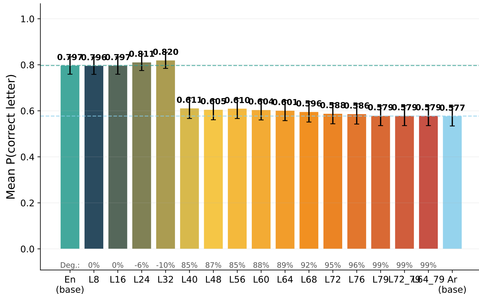
Llama-3.3-70B
