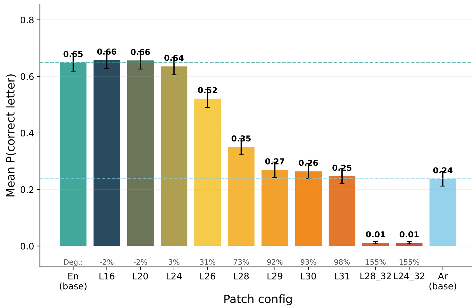
ALLaM-7B
