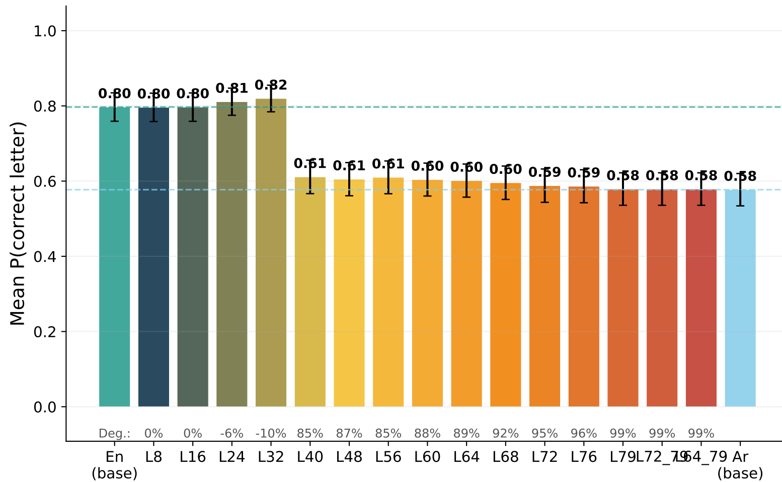
Llama-3.3-70B
