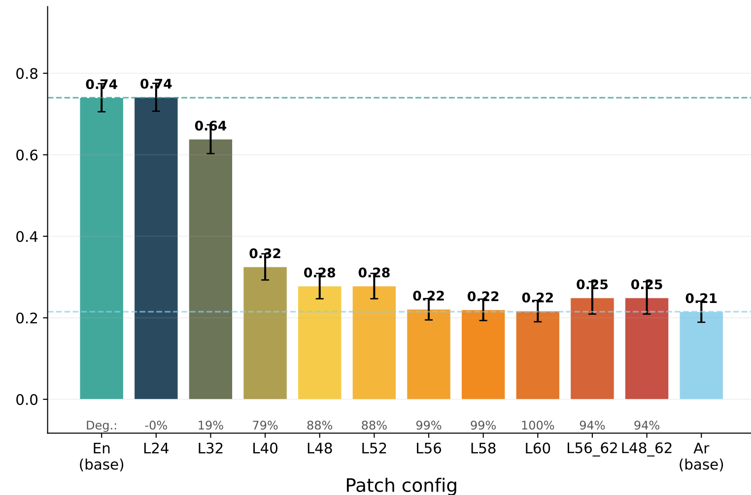
MedGemma-27B
