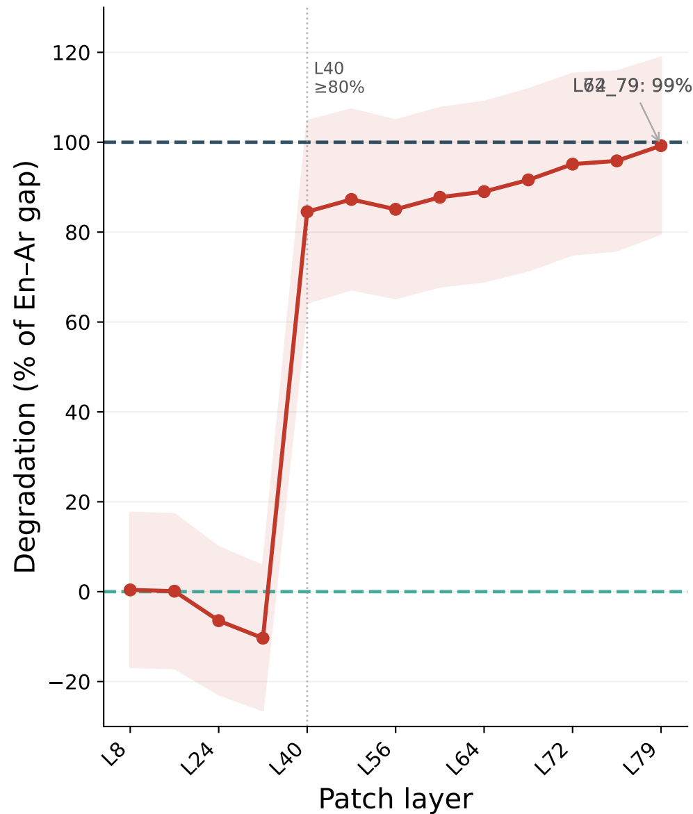
Llama-3.3-70B
