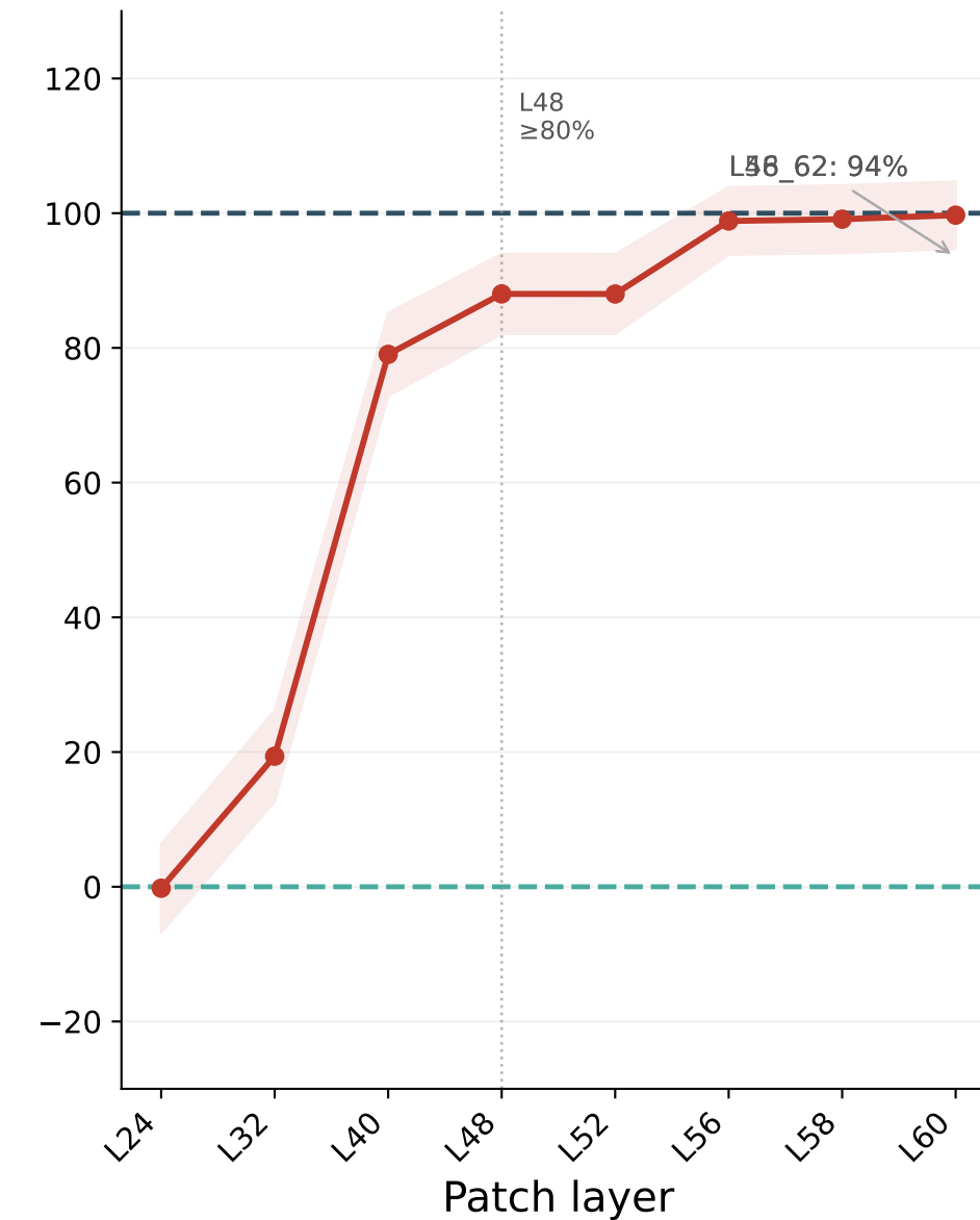
MedGemma-27B
