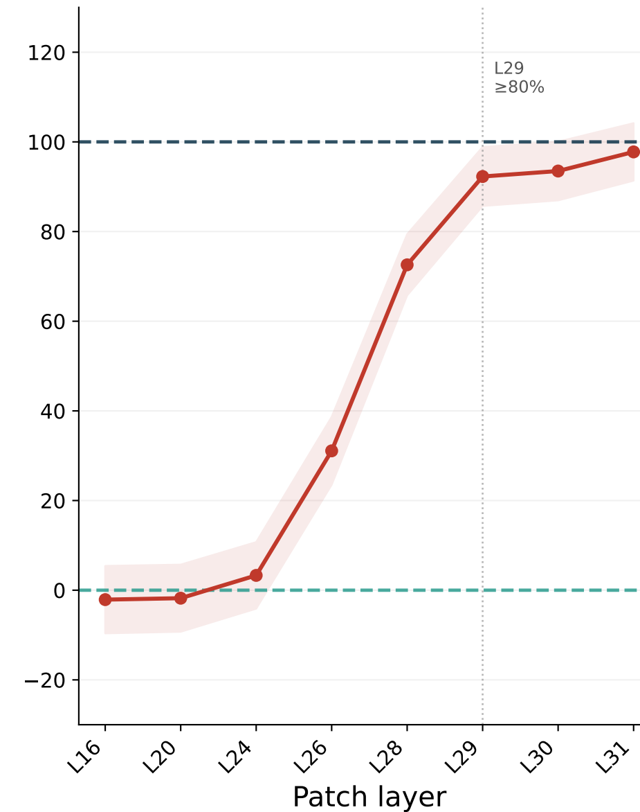
ALLaM-7B
