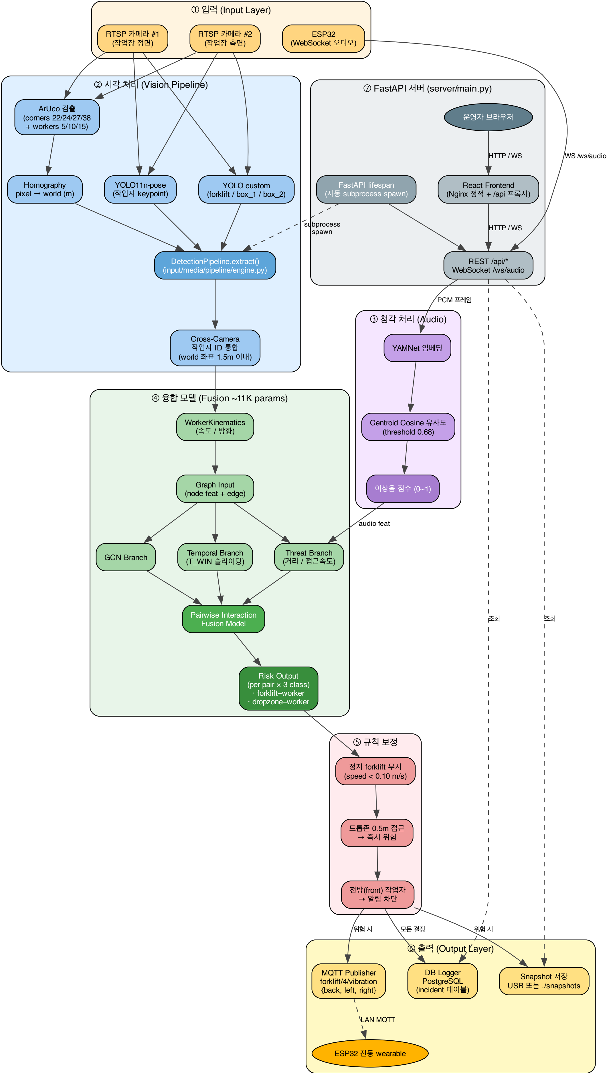
산업 안전 모니터링 시스템 — 전체 플로우
