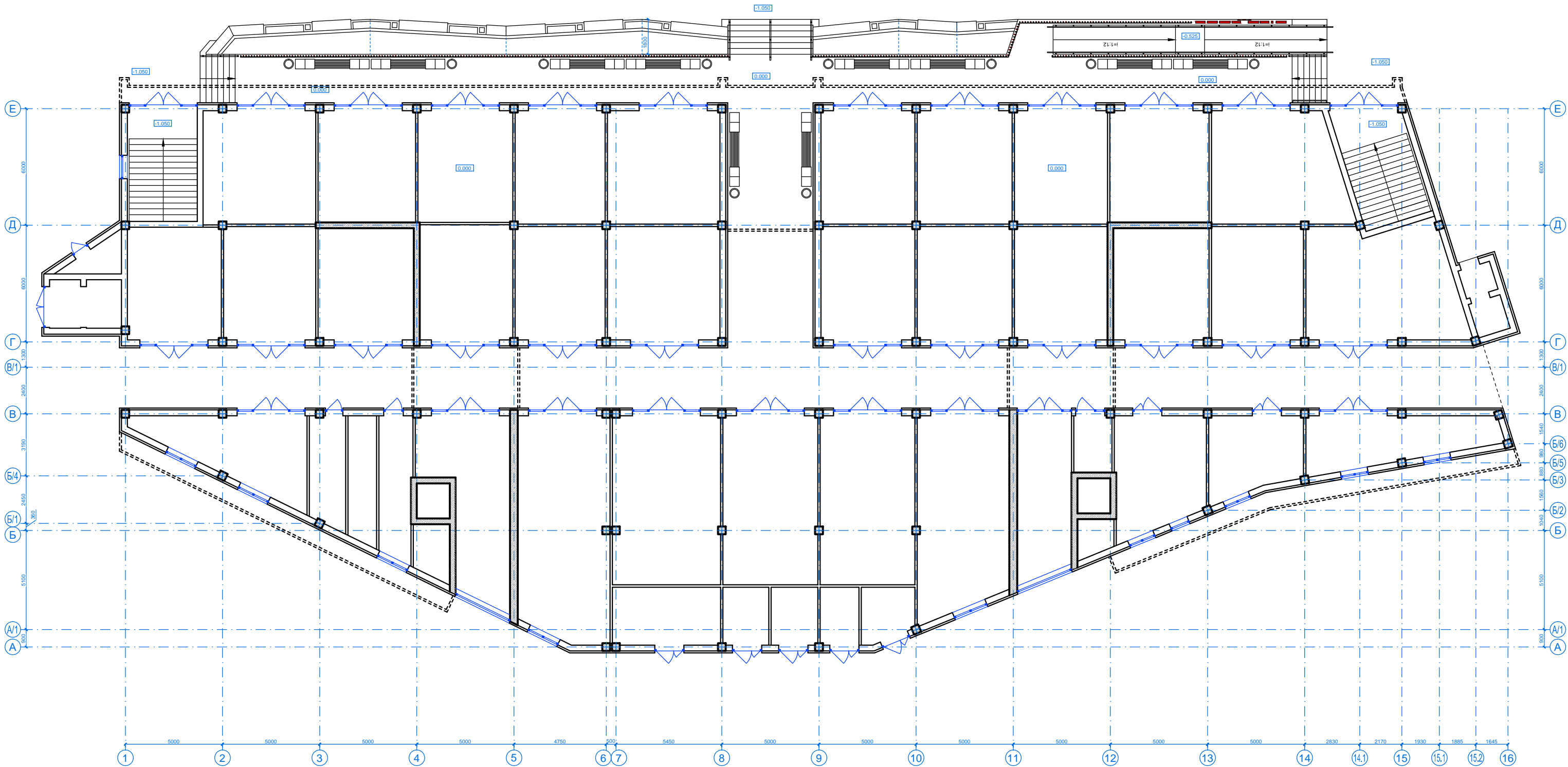
План 1 поверху М 1:100
