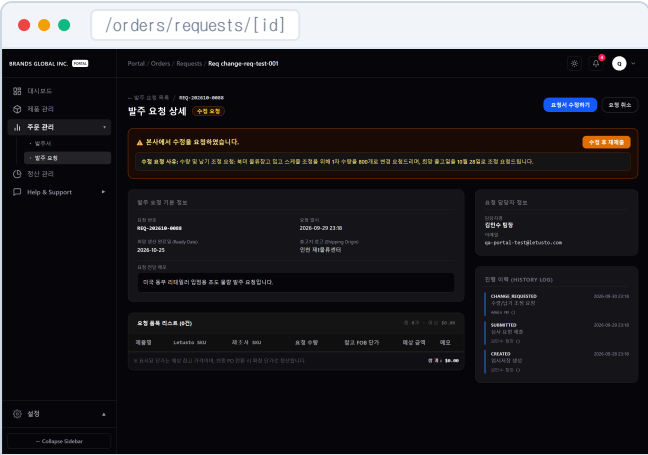
[그림 3-1] SCR-B-ORD-005 : MD 심사 및 수정 요청(CHANGE_REQUESTED) 상태 확인
