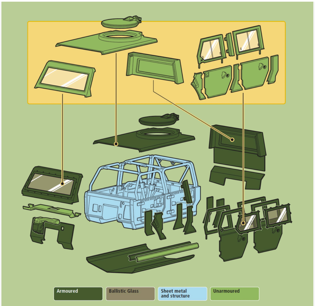
[그림 14] LMV의 모듈러식 방탄구성(출처 : IVECO)
