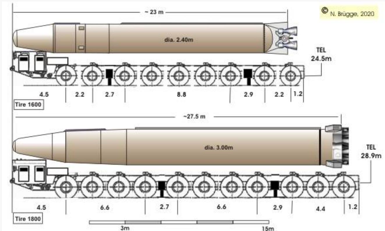
[그림 4] 화성-15호, 화성-16호 크기 비교(출처 : http://www.b14643.de/ )
