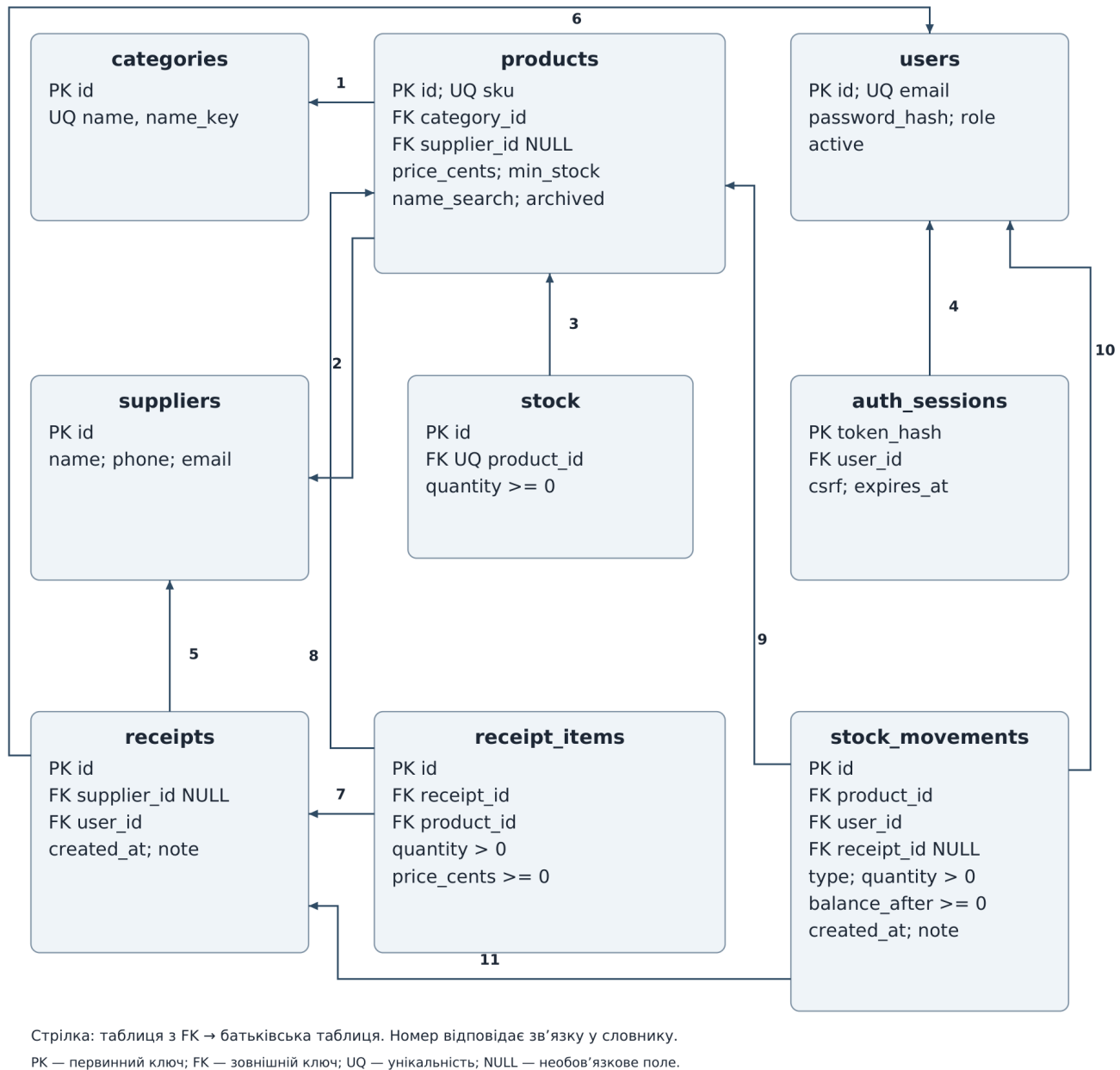
Рисунок 4. ER схема з напрямком FK до батьківської таблиці.
