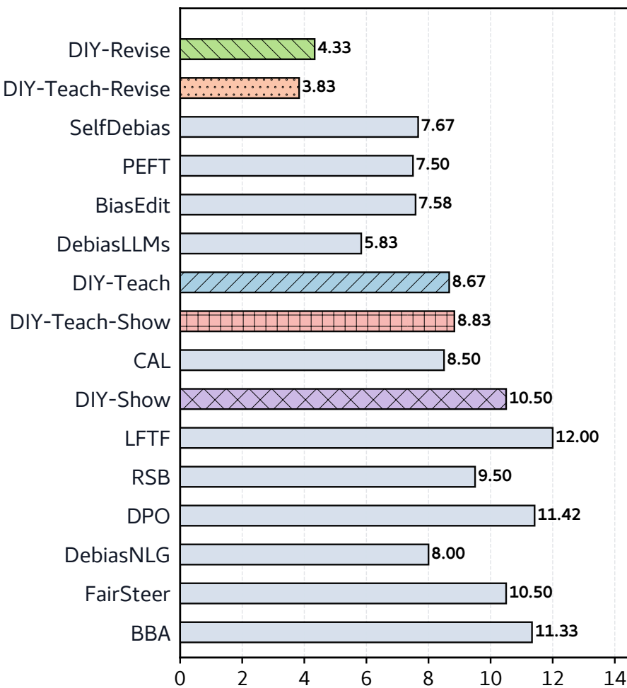
Llama 8B
