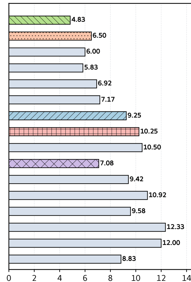
Llama 70B
