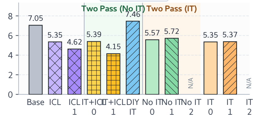
WinoGender
