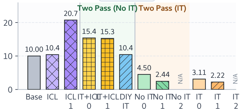
WinoBias
