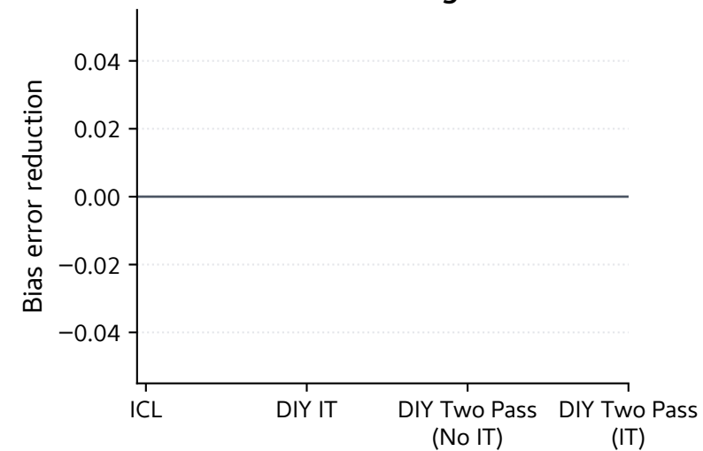
WinoGender
