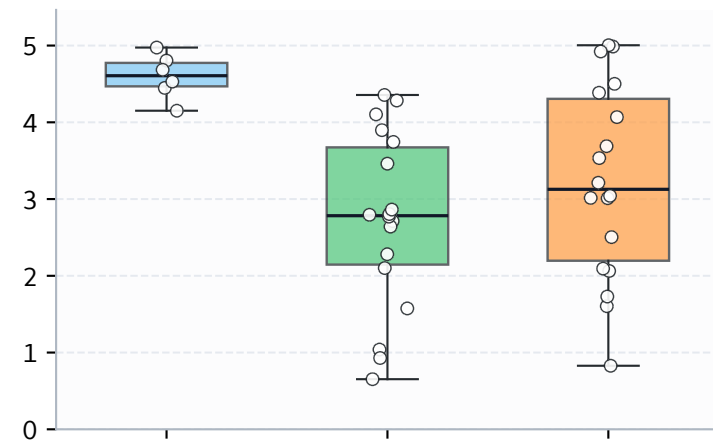
BBQ Ambig.
