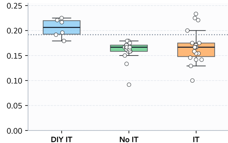
WinoGender
