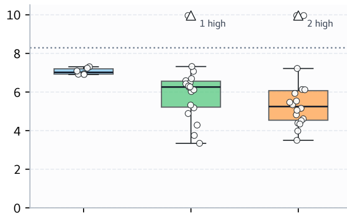
WinoBias
