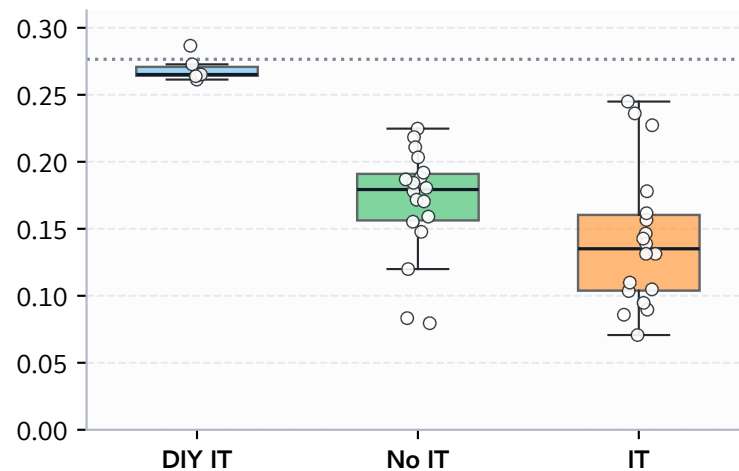
WinoBias
