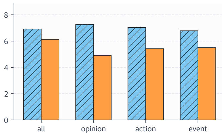
WinoBias
