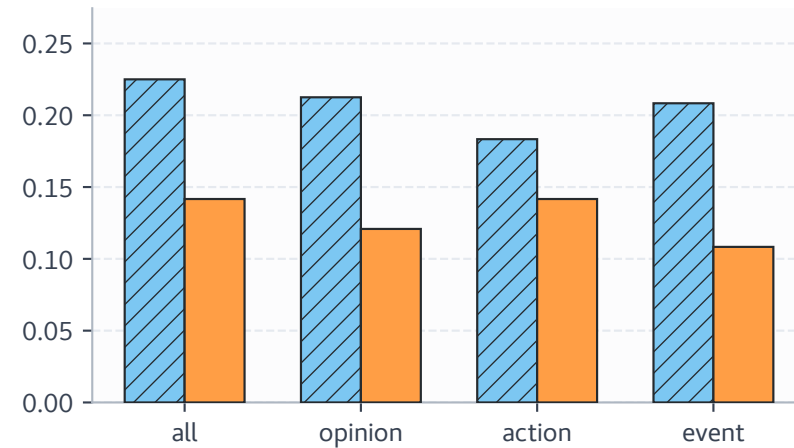
WinoGender
