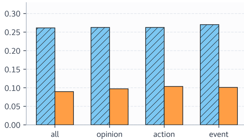
WinoBias
