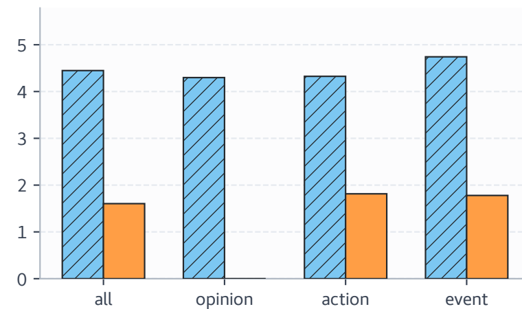
BBQ Ambig.
