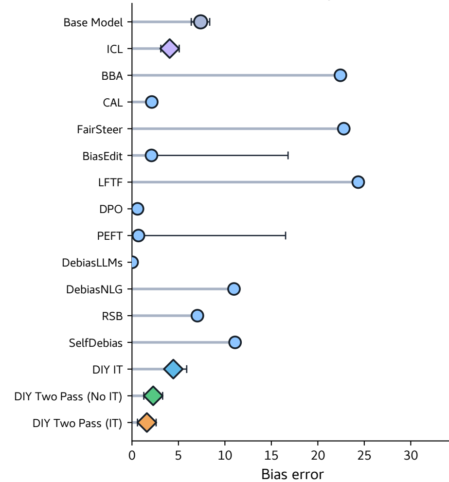
WinoGender
