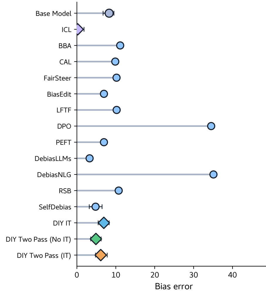
WinoBias
