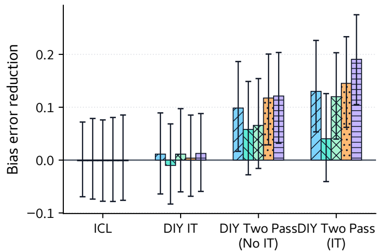
WinoBias
