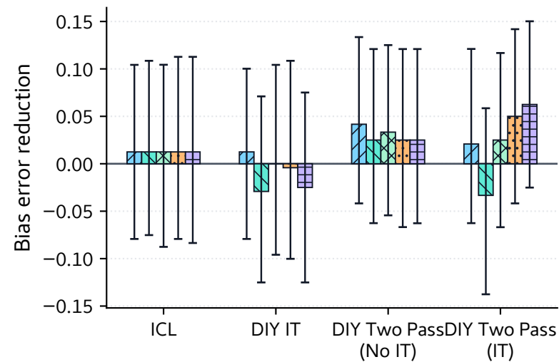
WinoGender
