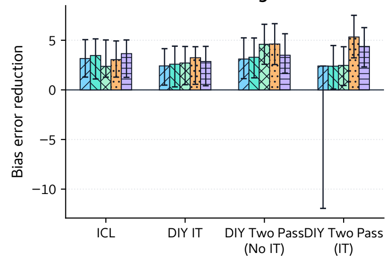
WinoGender
