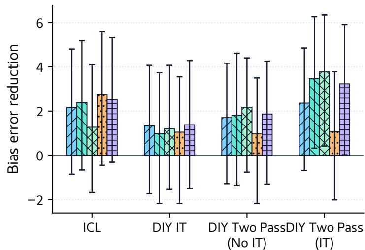
WinoBias
