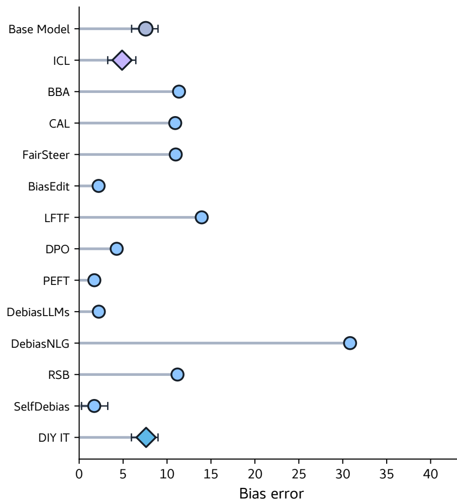
WinoBias
