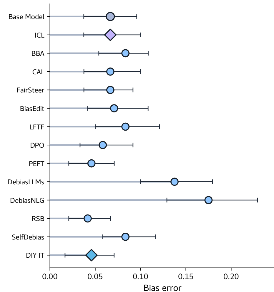
WinoGender
