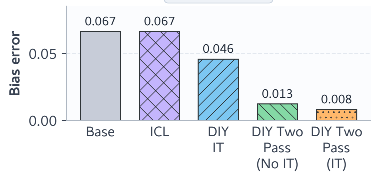
WinoGender
