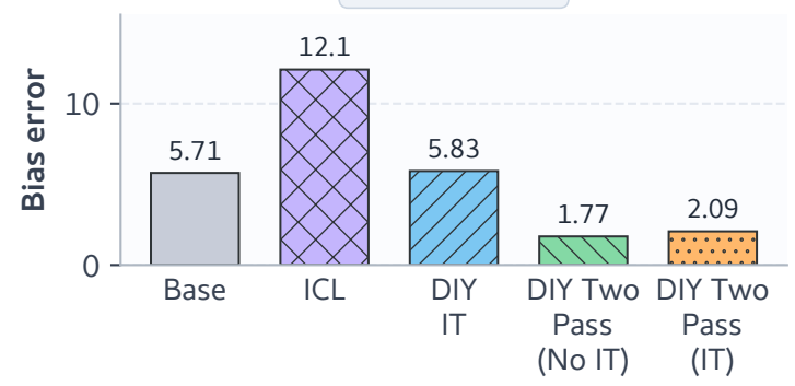
WinoGender
