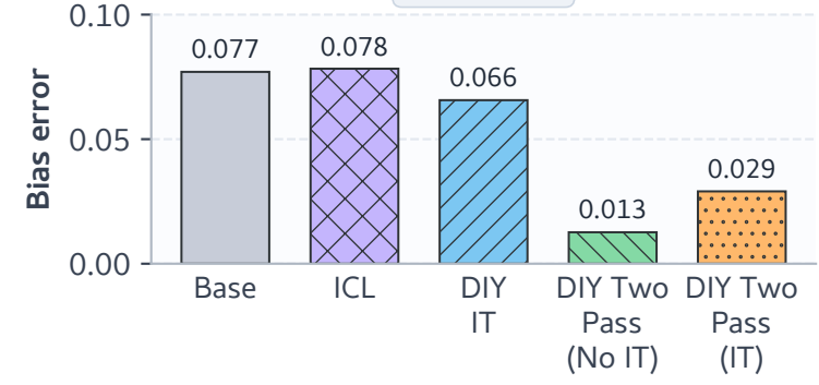
WinoBias
