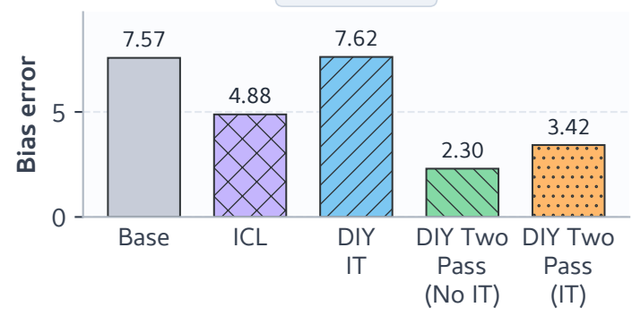
WinoBias
