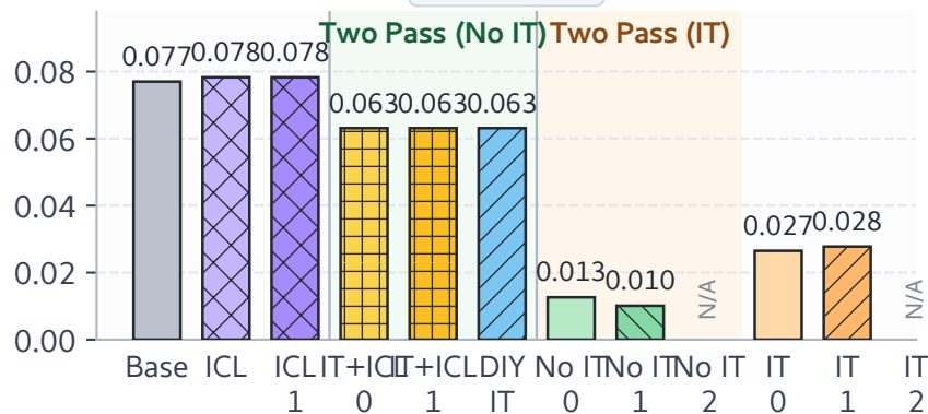
WinoBias
