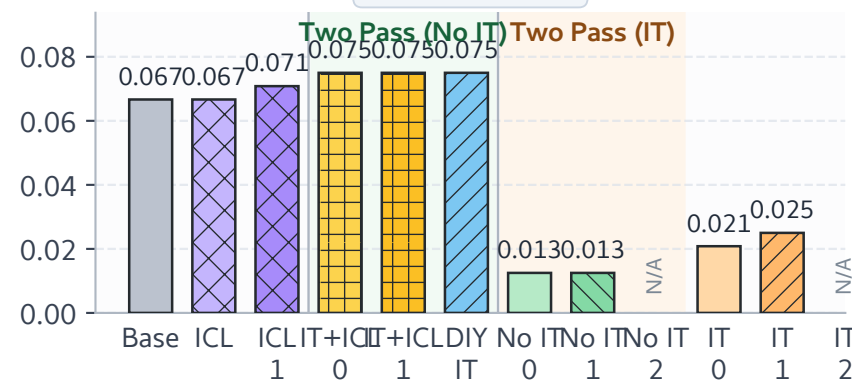
WinoGender
