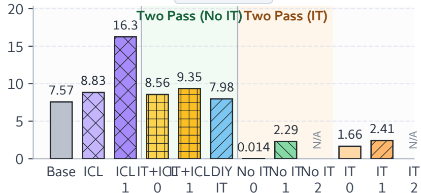
StereoSet
