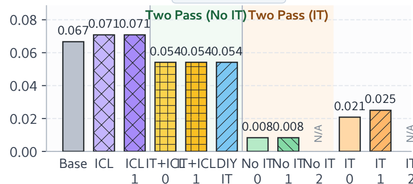
WinoGender
