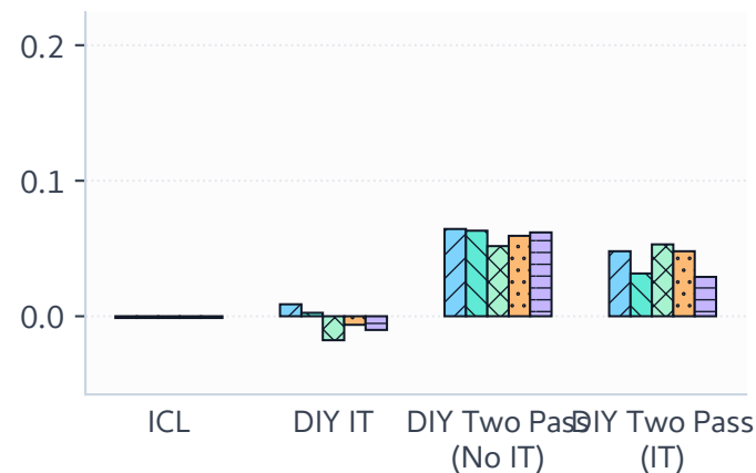
WinoBias
