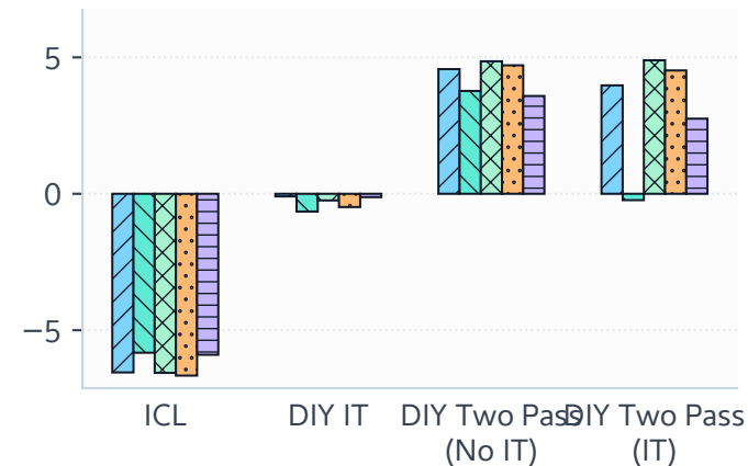
WinoGender
