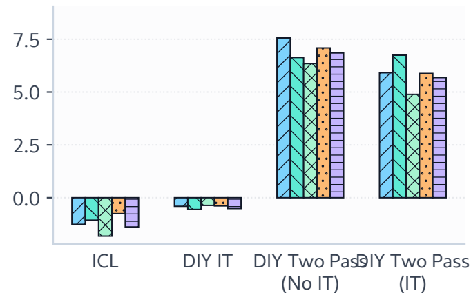
WinoBias
