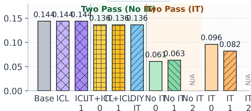
WinoBias
