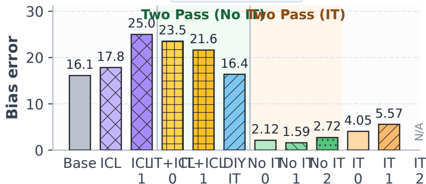
CrowS-Pairs
