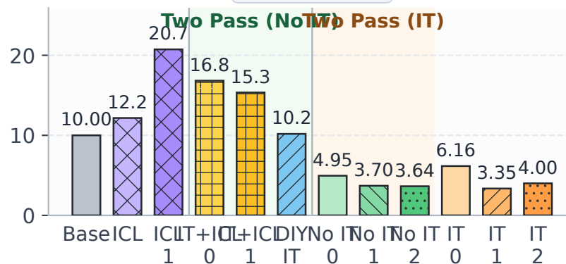
StereoSet
