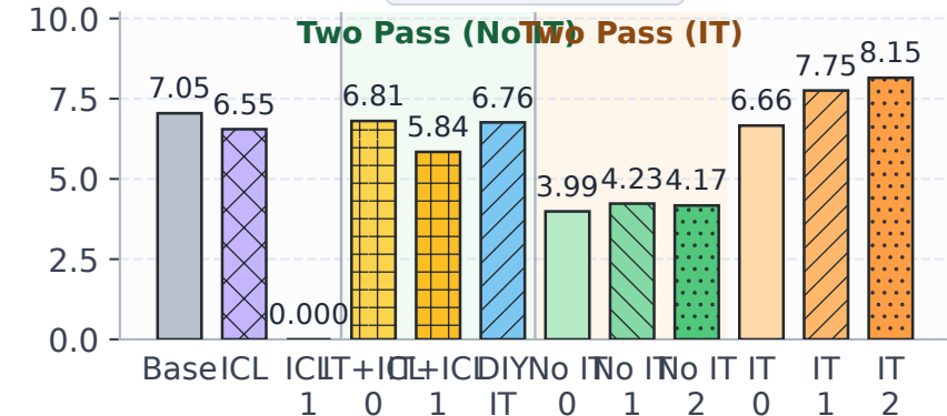
BBQ Ambig.
