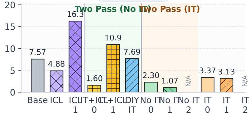
StereoSet
