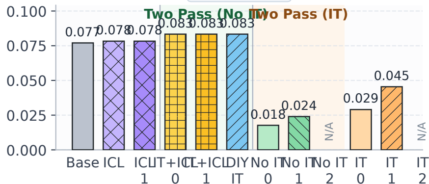
WinoBias
