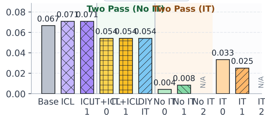
WinoGender
