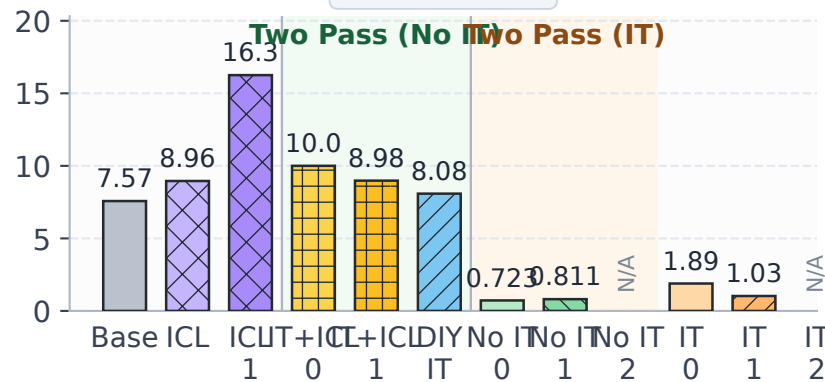
StereoSet
