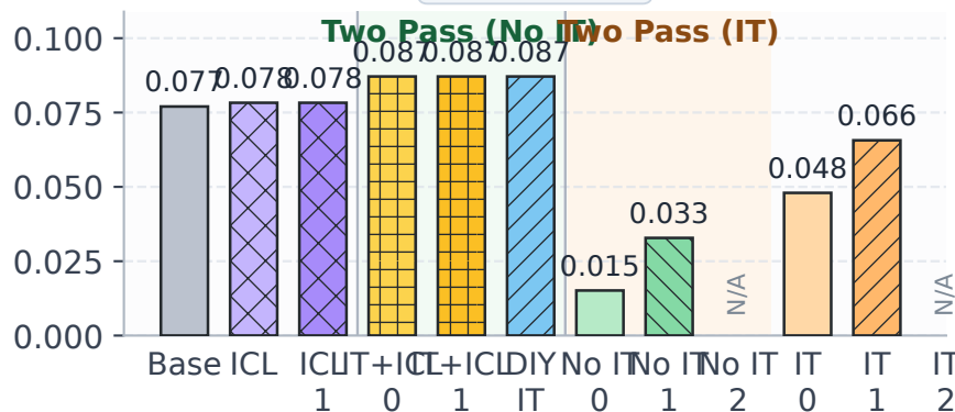
WinoBias
