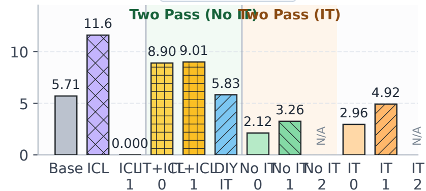
BBQ Ambig.
