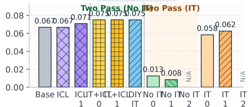
WinoGender
