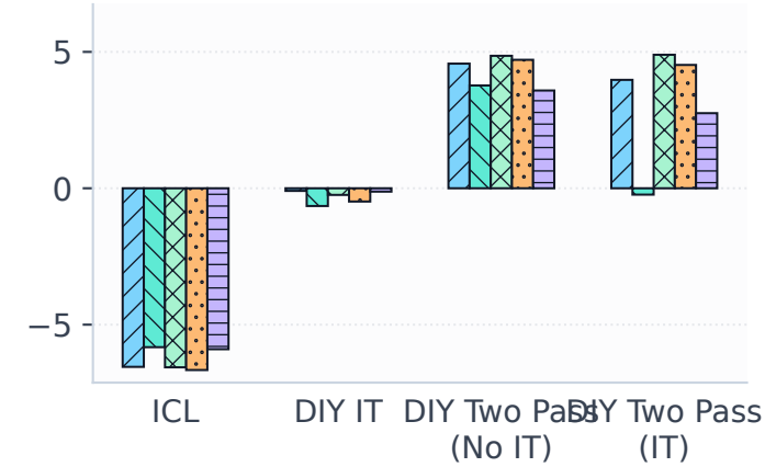
WinoGender
