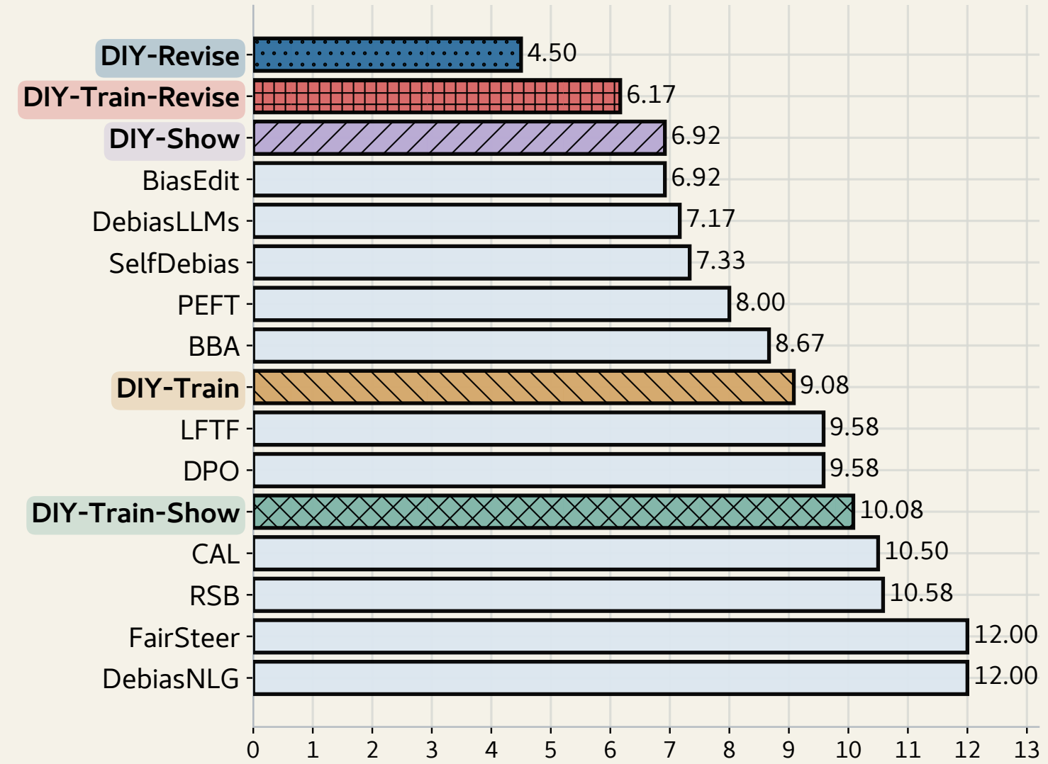
Llama 70B
