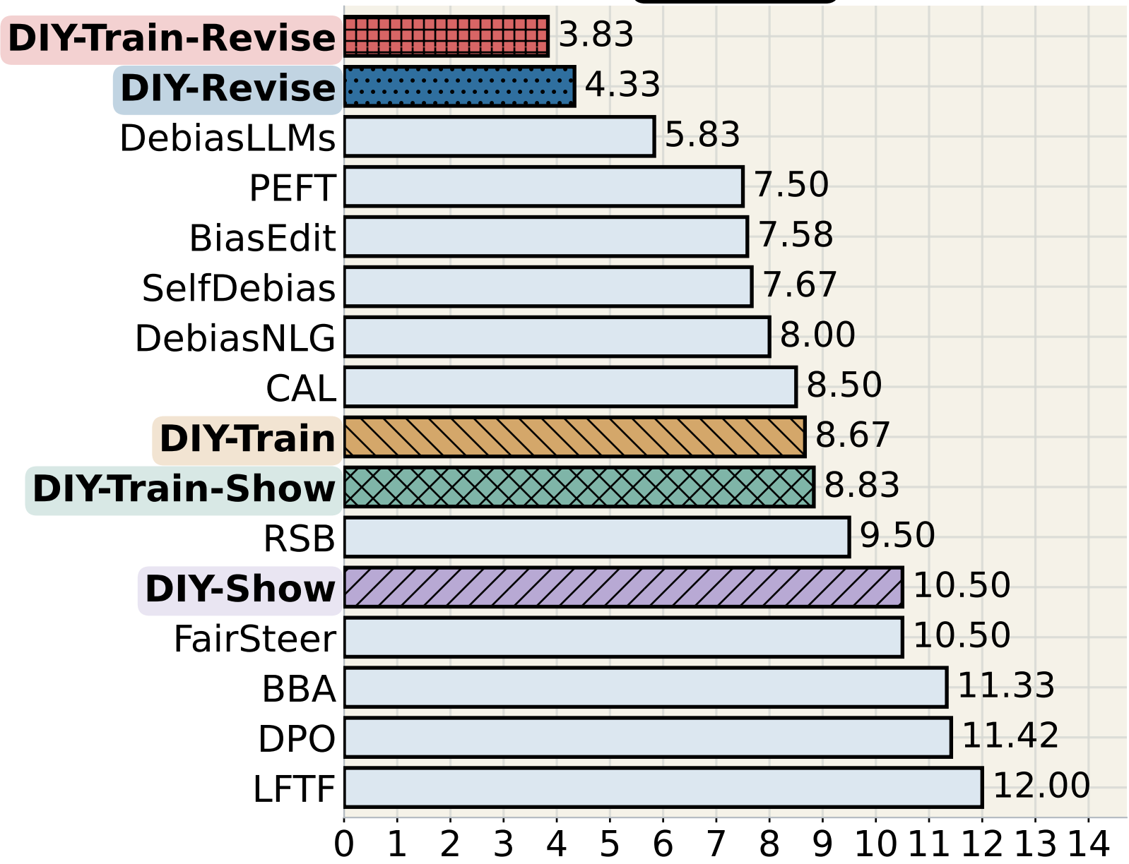
Llama 8B
