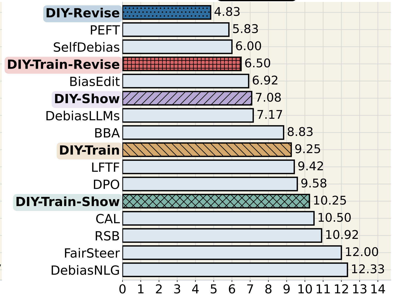
Llama 70B
