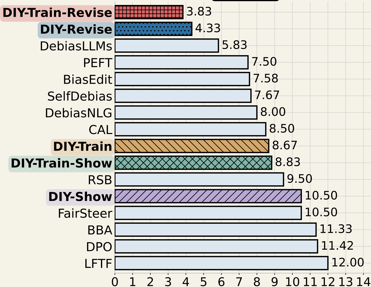
Llama 8B
