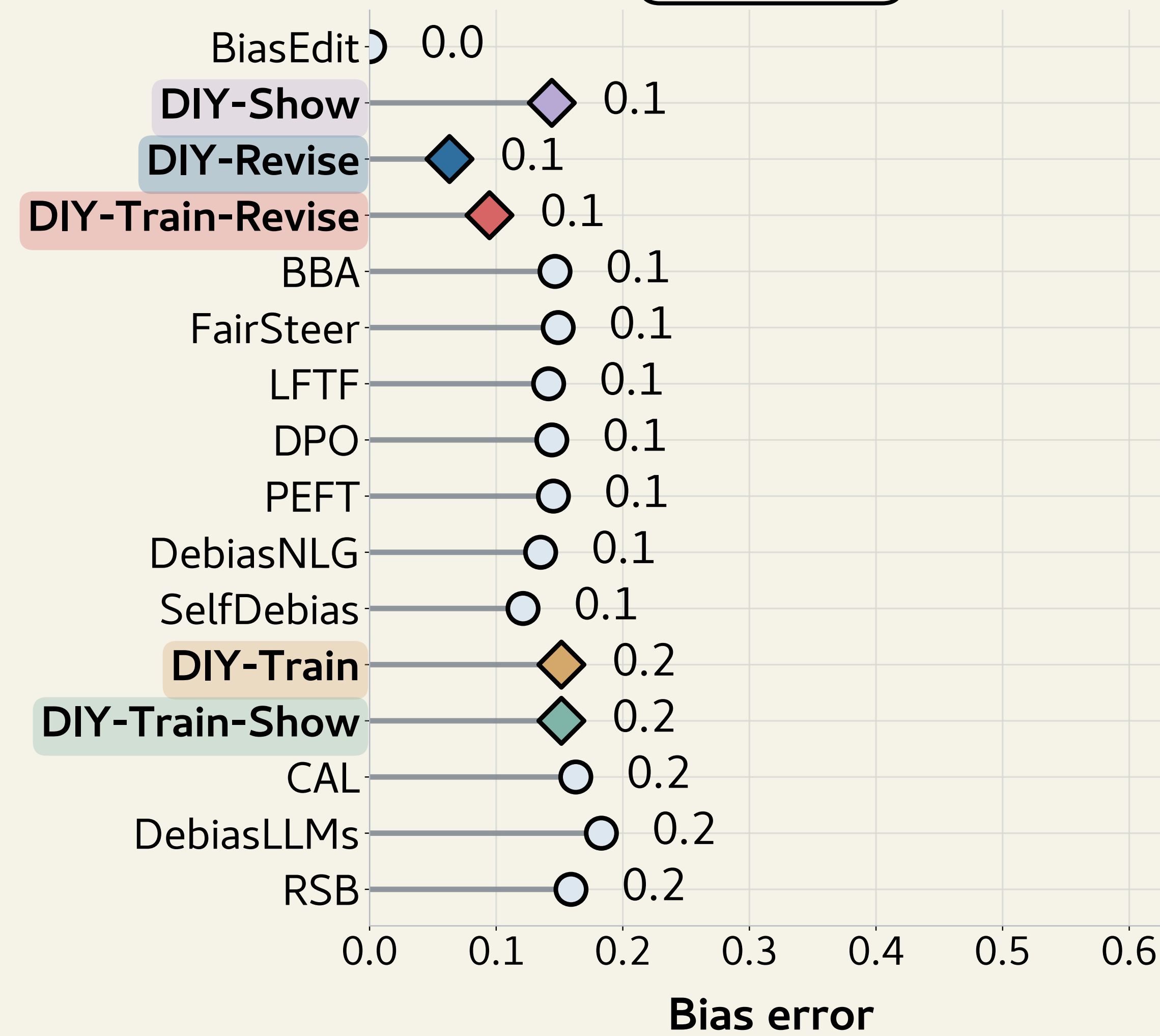
WinoBias
