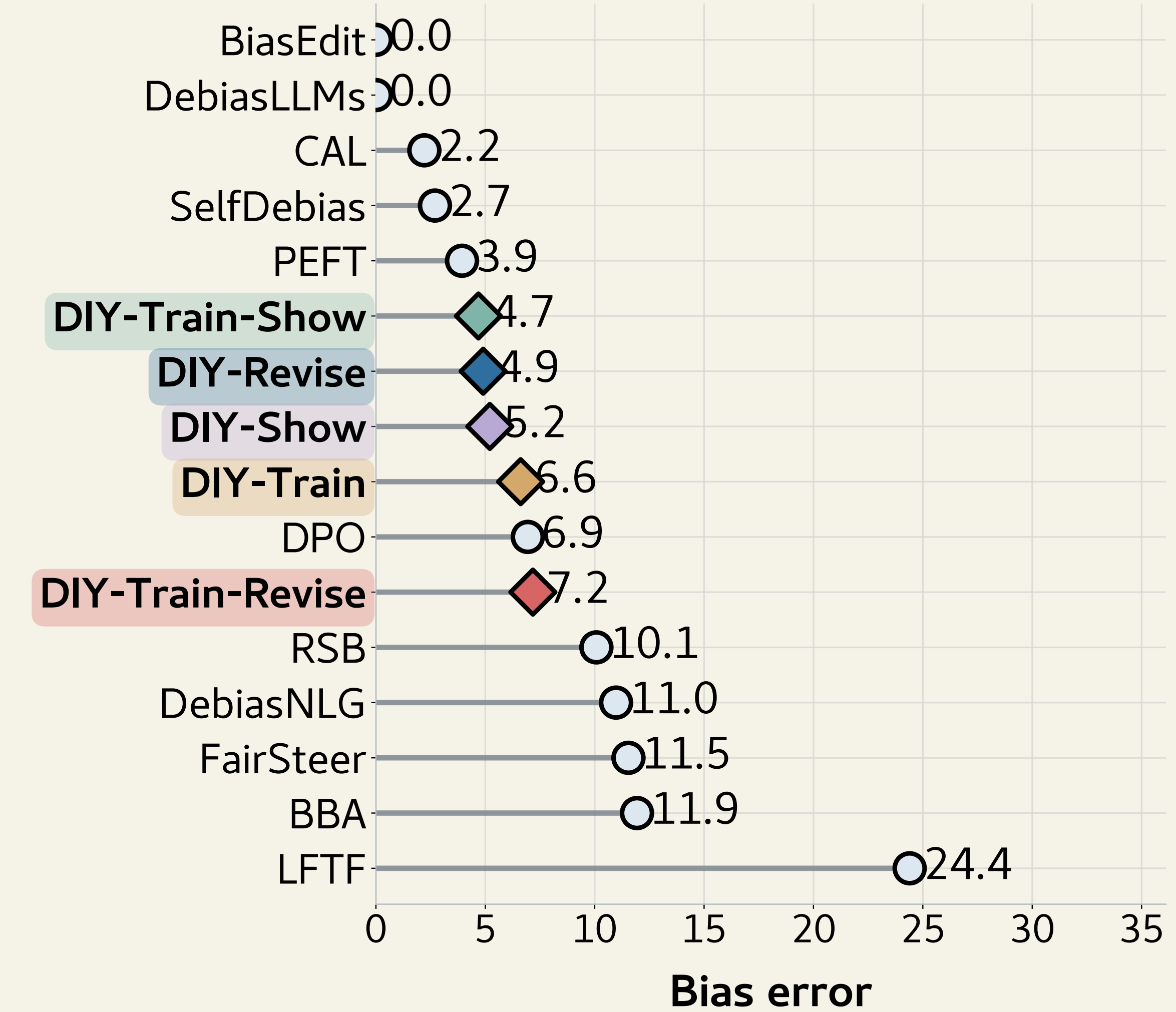
BBQ Ambig.
