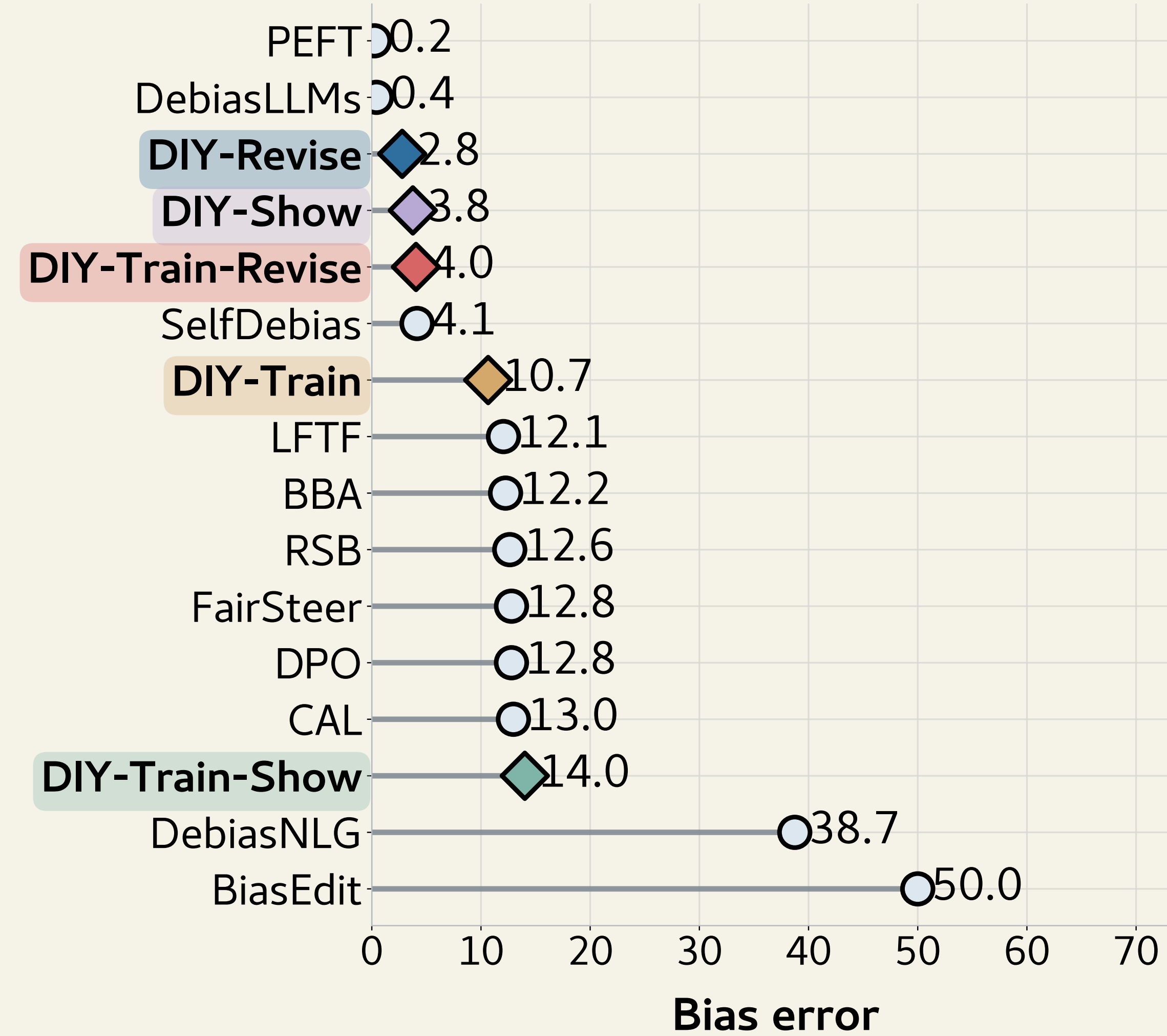
StereoSet
