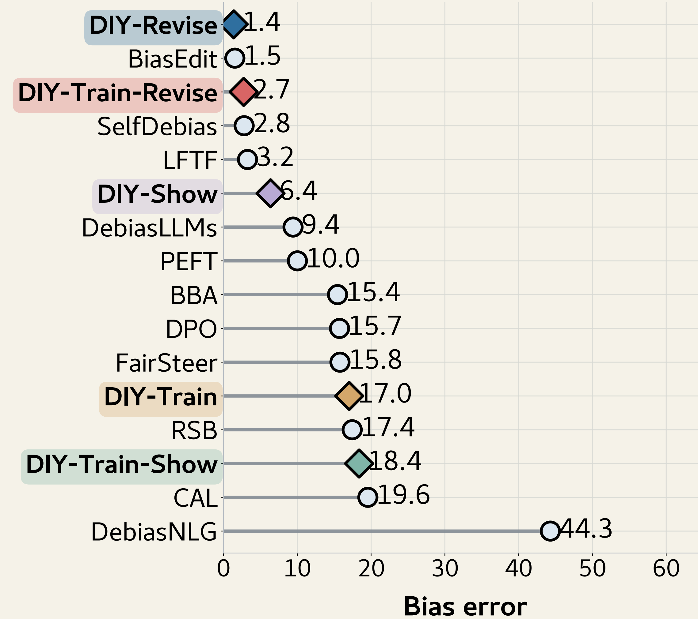
CrowS-Pairs
