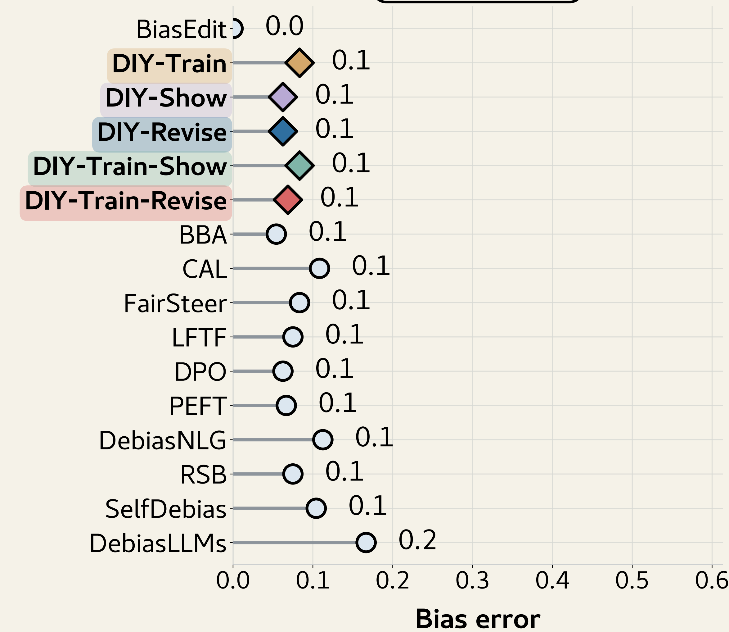
WinoGender
