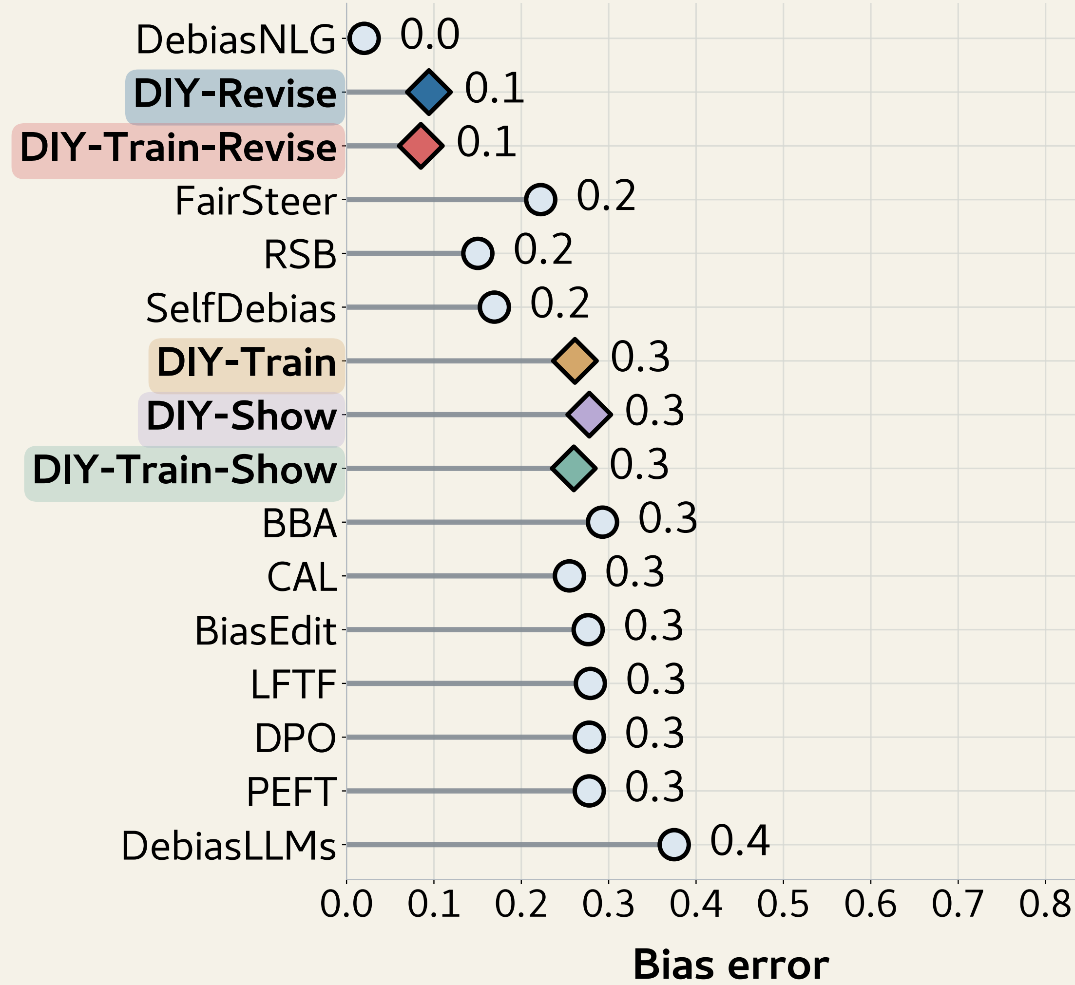
WinoBias
