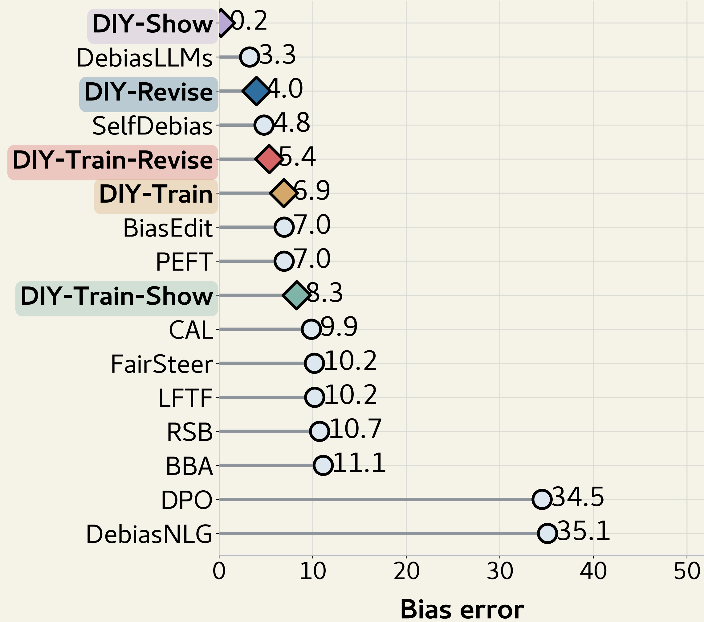
StereoSet
