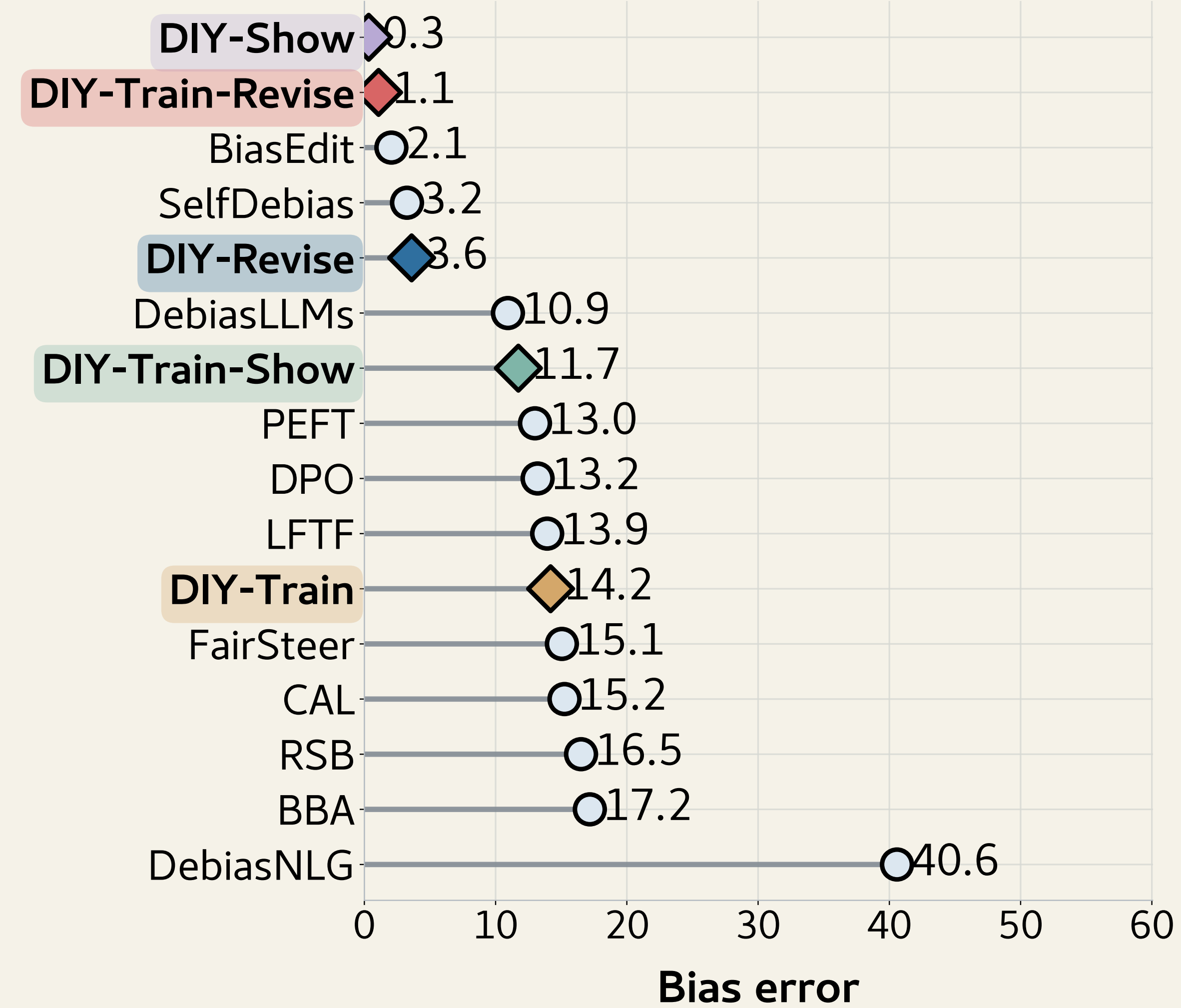
CrowS-Pairs
