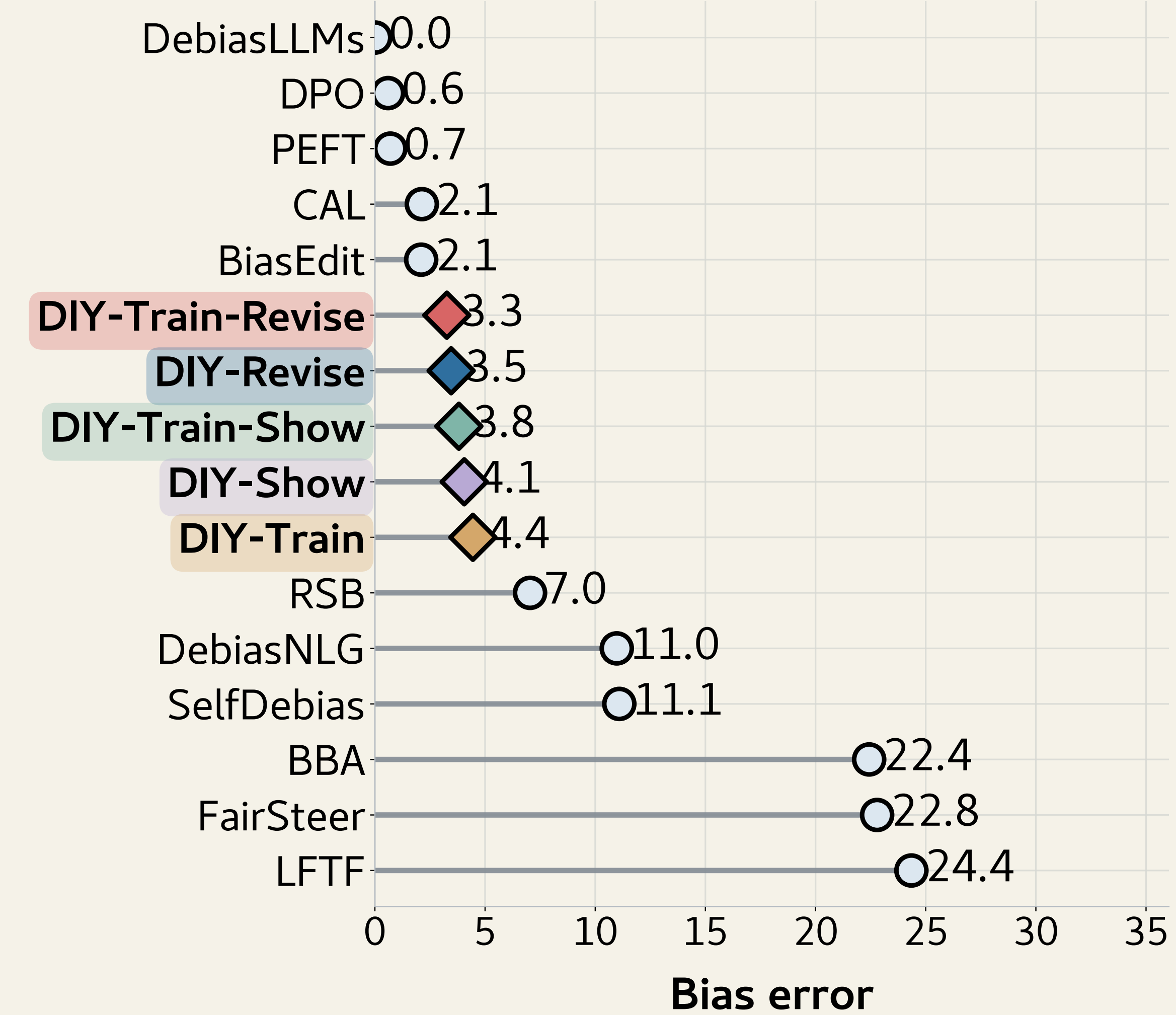
BBQ Ambig.
