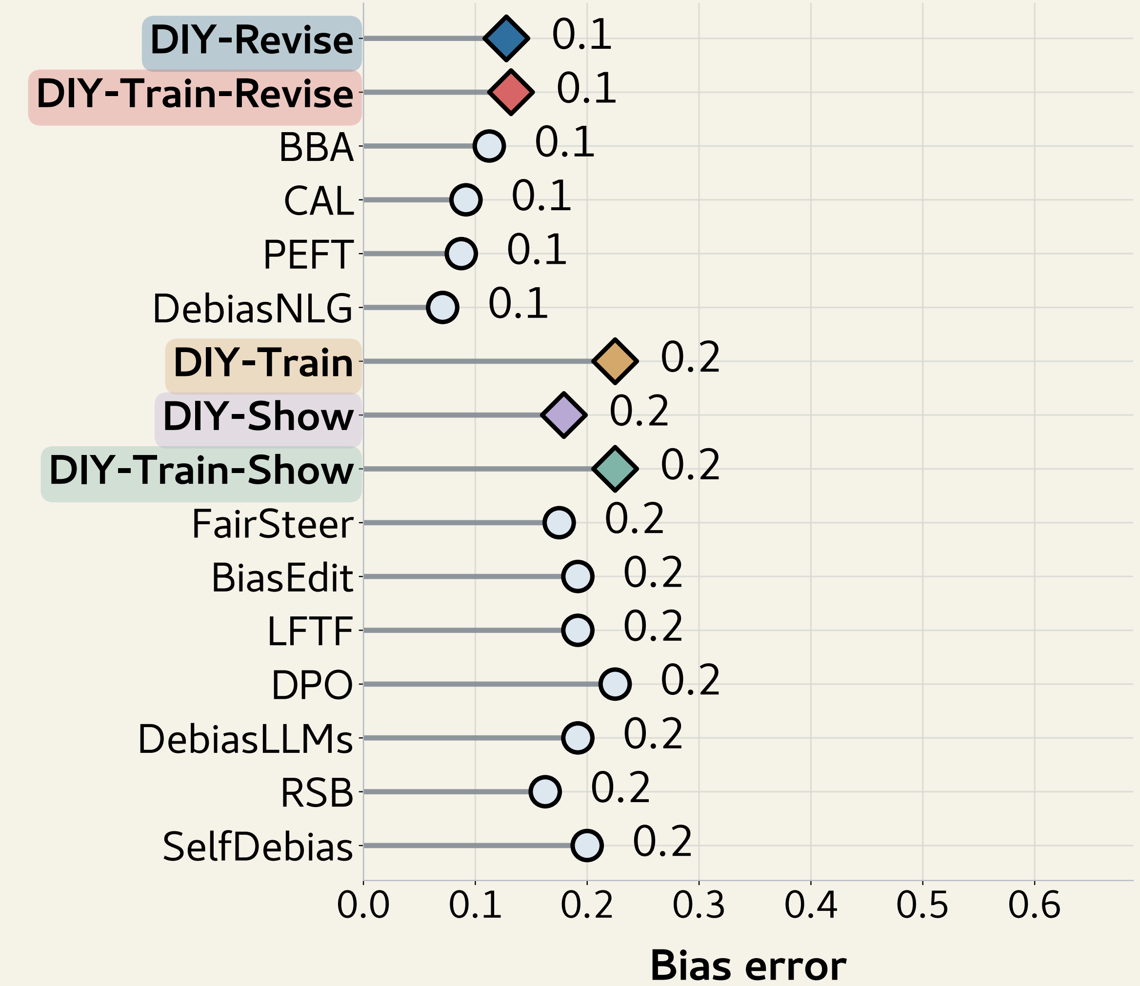
WinoGender
