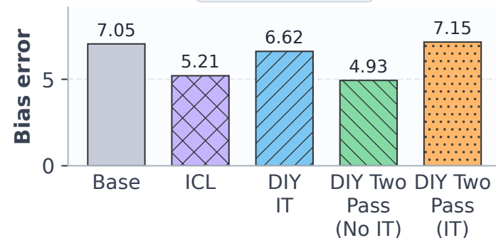
BBQ Ambig.
