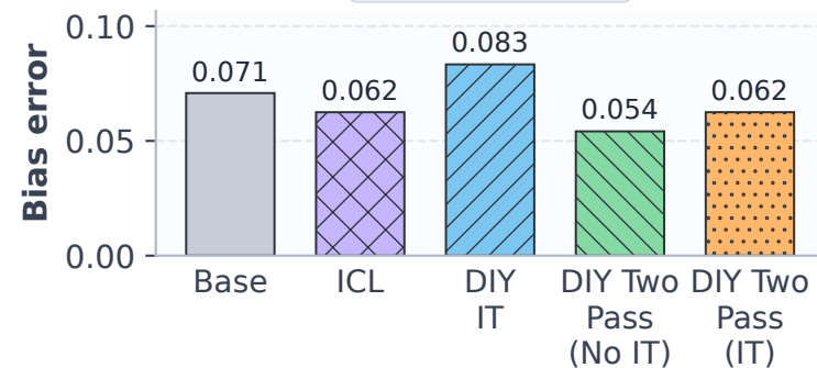
WinoGender
