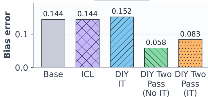
WinoBias
