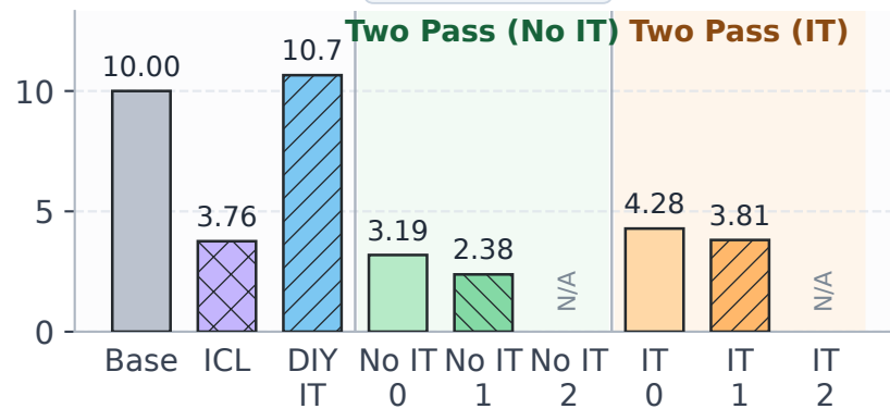
StereoSet
