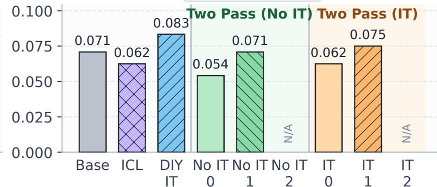
WinoGender
