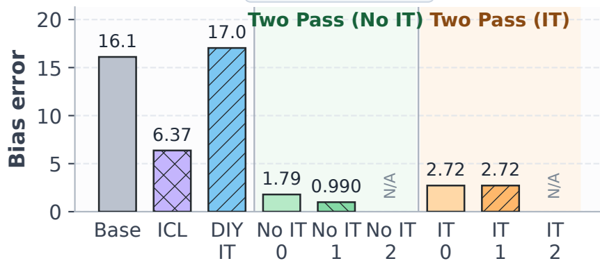
CrowS-Pairs
