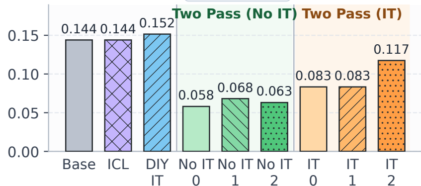
WinoBias
