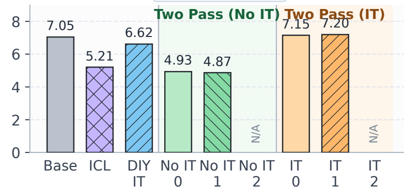
BBQ Ambig.
