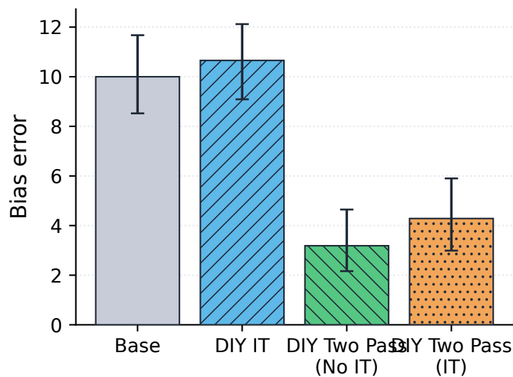
WinoBias
