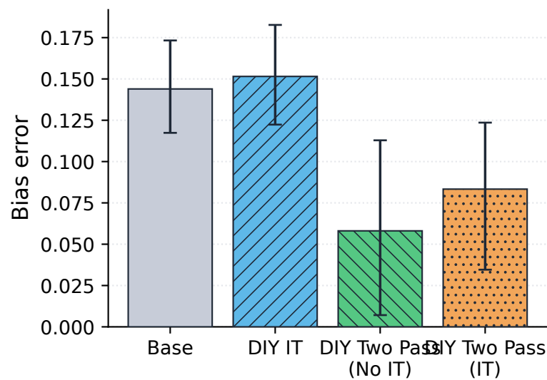
WinoBias
