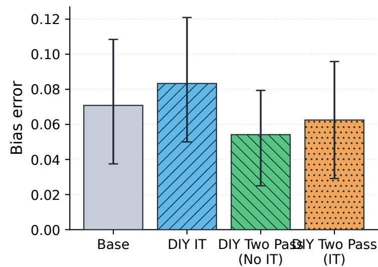
WinoGender
