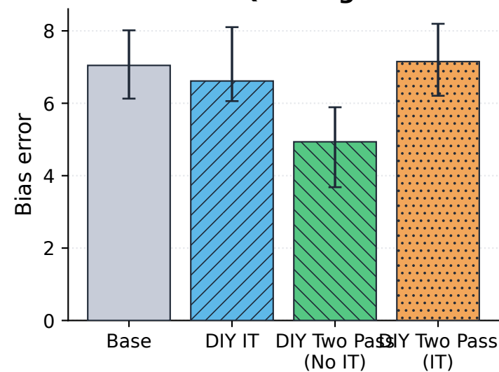
WinoGender
