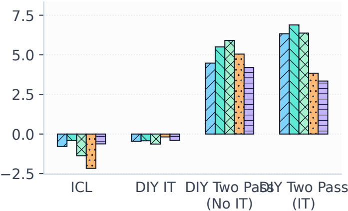
WinoBias
