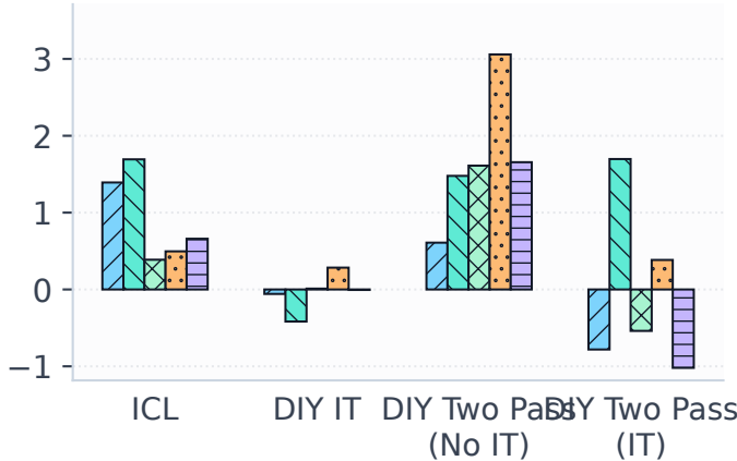
WinoGender
