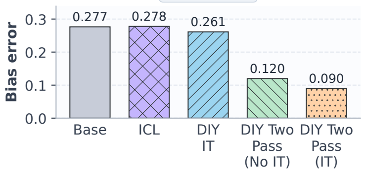
WinoBias
