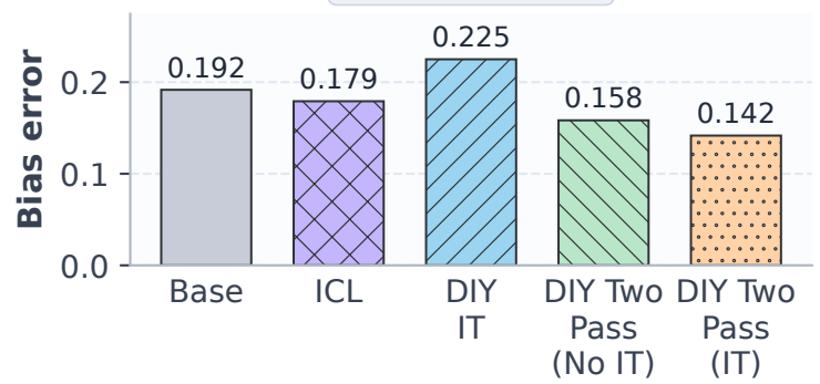
WinoGender
