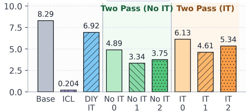
StereoSet
