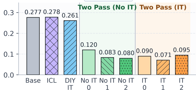
WinoBias
