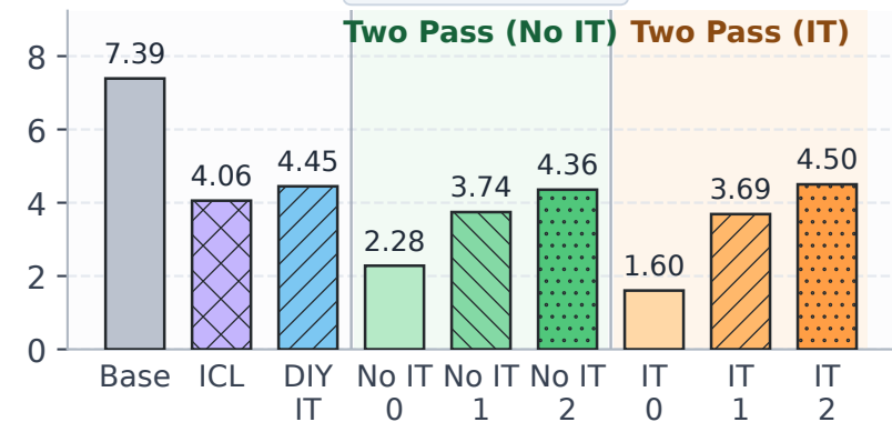
BBQ Ambig.
