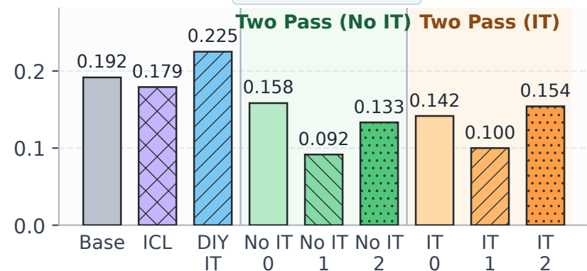
WinoGender
