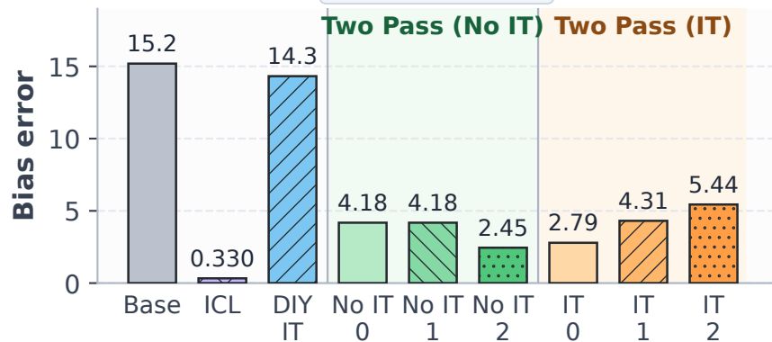
CrowS-Pairs
