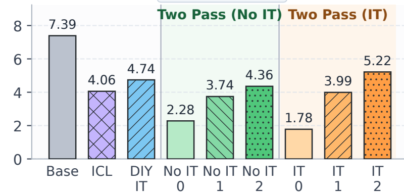
BBQ Ambig.
