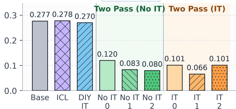
WinoBias
