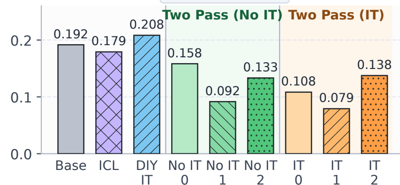
WinoGender
