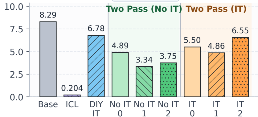
StereoSet
