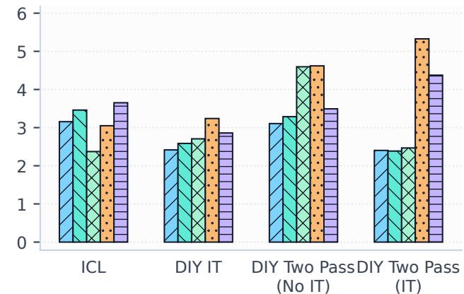
WinoGender
