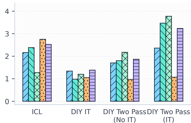
WinoBias
