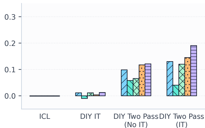
WinoBias
