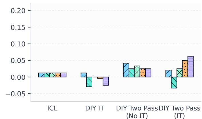
WinoGender
