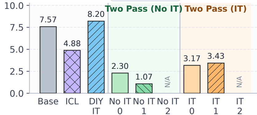
StereoSet
