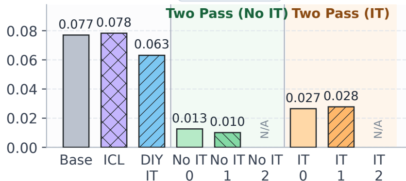
WinoBias
