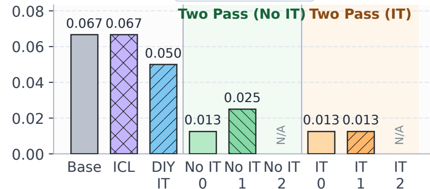
WinoGender
