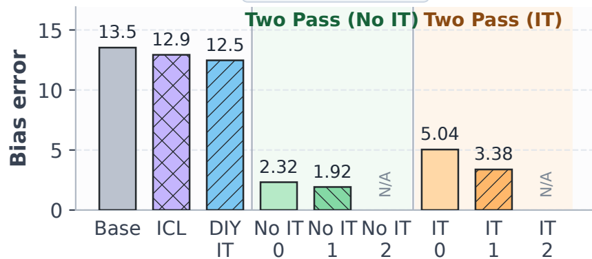
CrowS-Pairs
