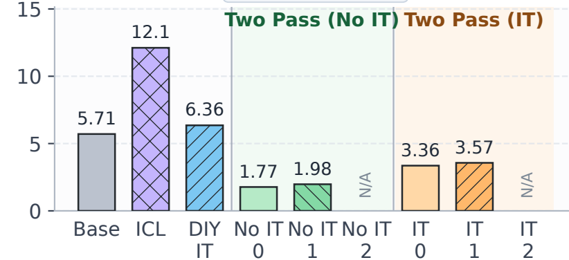
BBQ Ambig.
