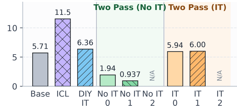
BBQ Ambig.
