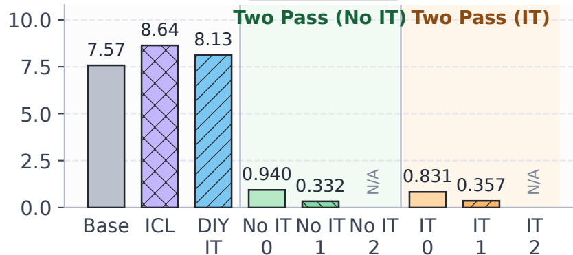
StereoSet
