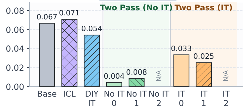
WinoGender
