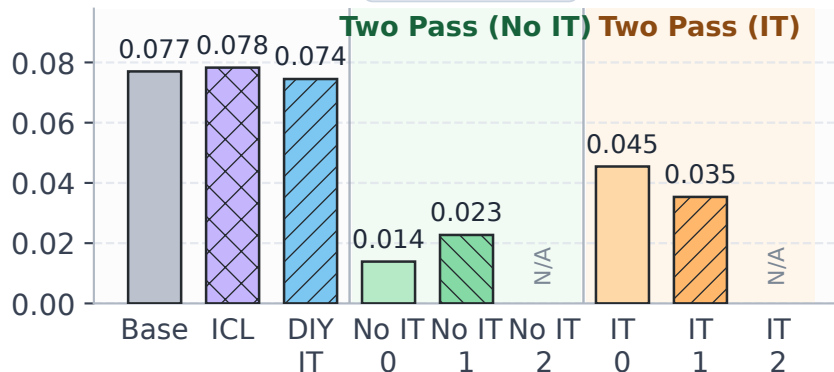
WinoBias
