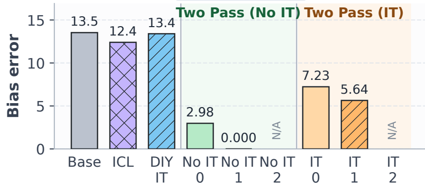
CrowS-Pairs
