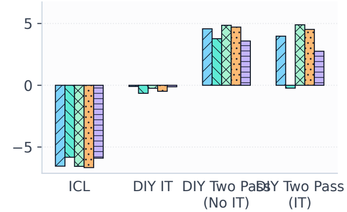
WinoGender
