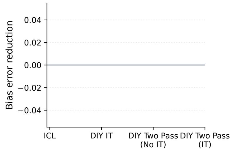
WinoBias
