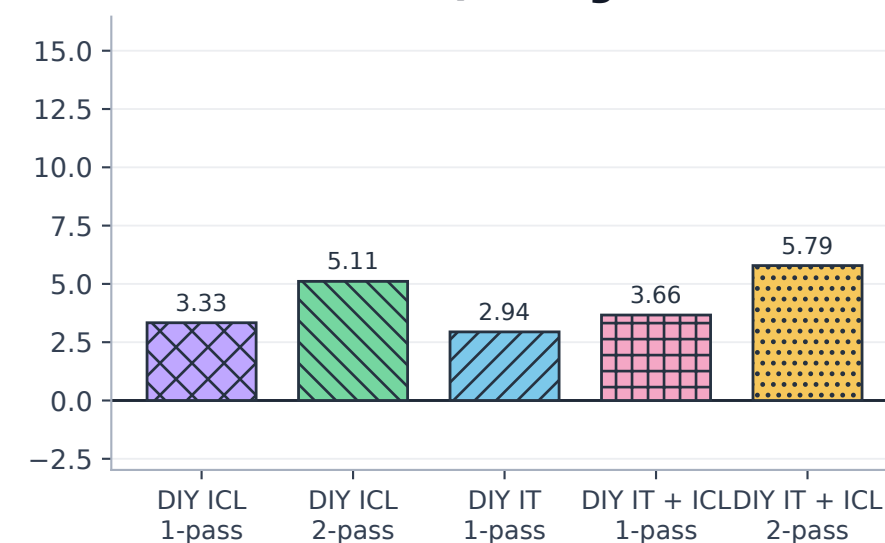
BBQ Ambig.
