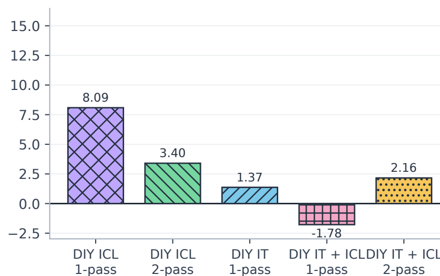
StereoSet
