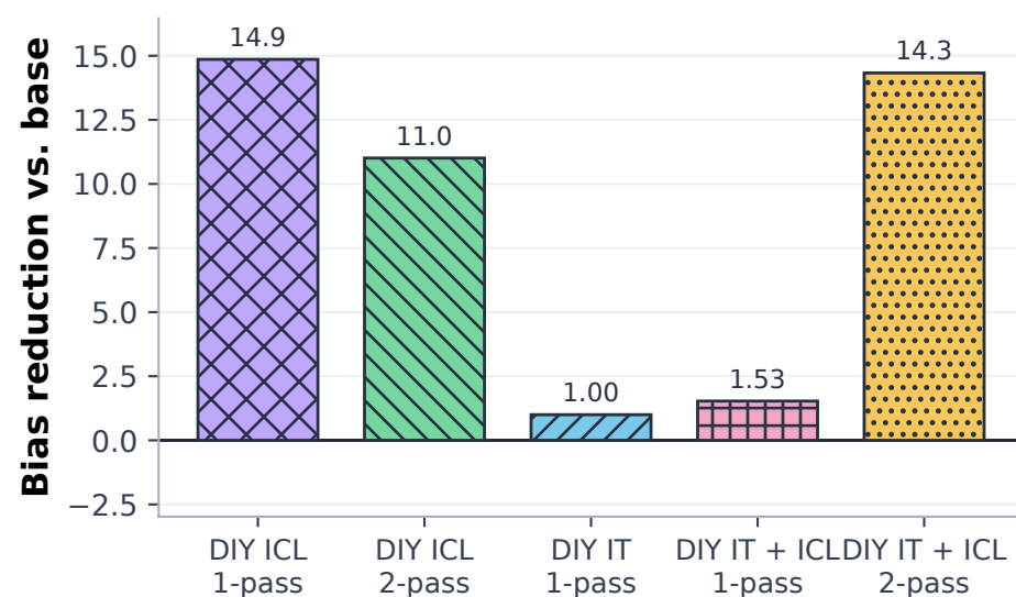
CrowS-Pairs
