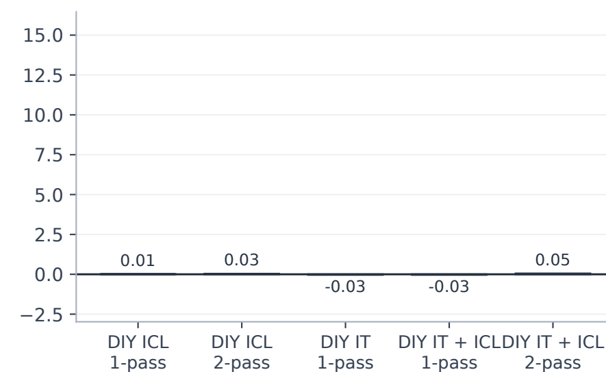
WinoGender
