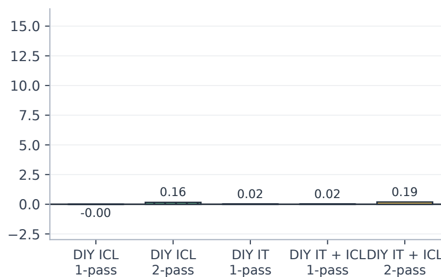
WinoBias
