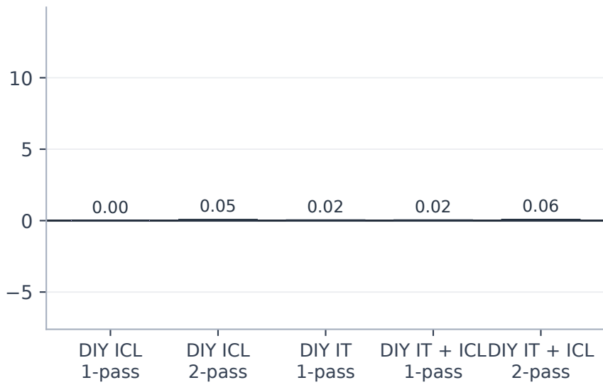
WinoGender
