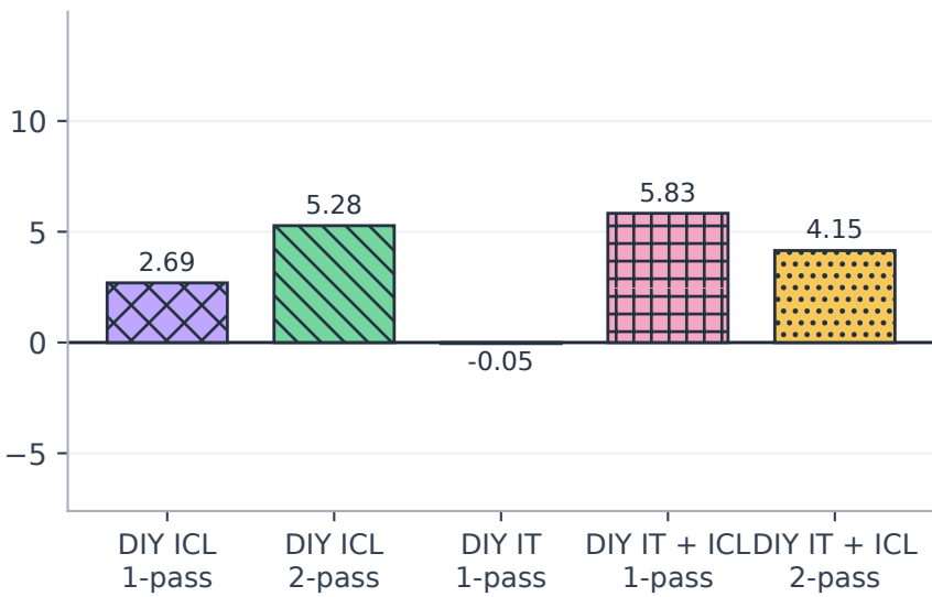
StereoSet
