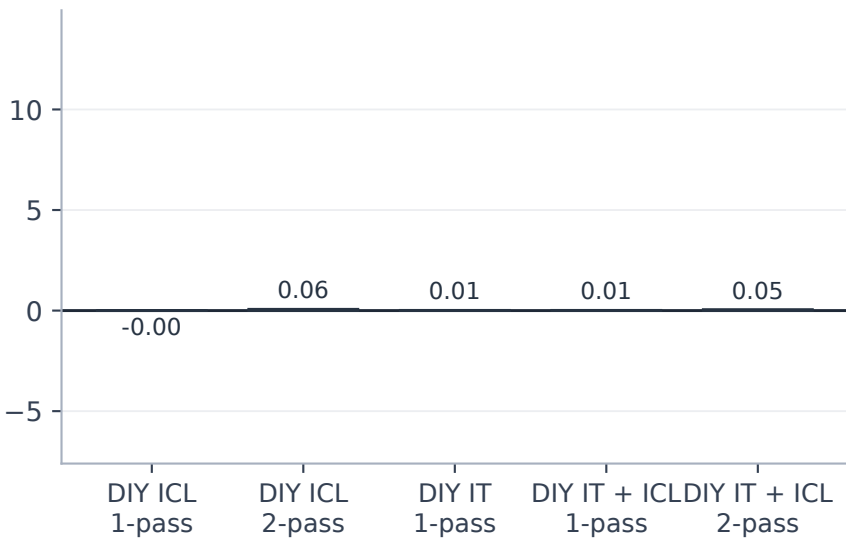
WinoBias
