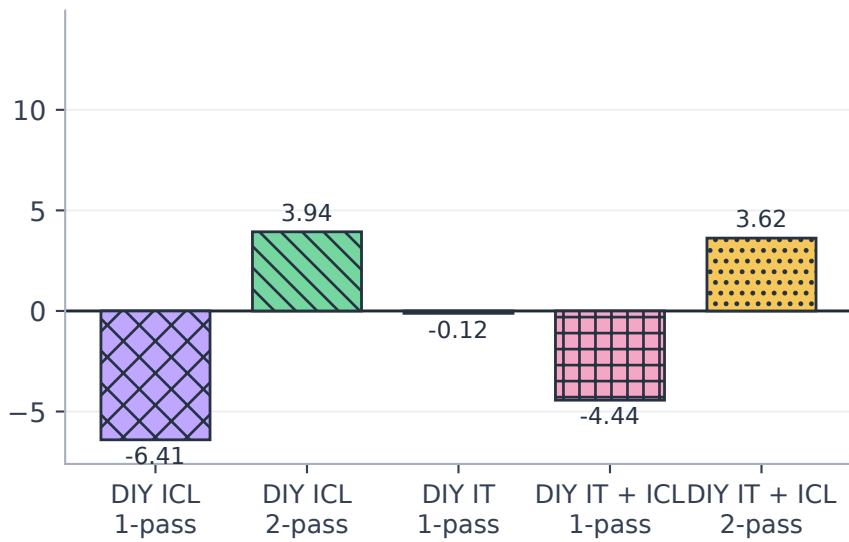
BBQ Ambig.
