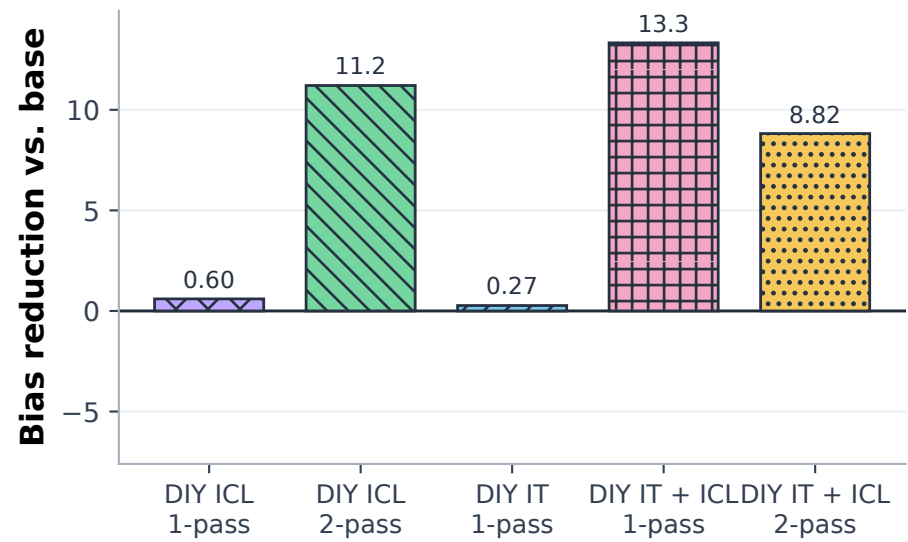
CrowS-Pairs
